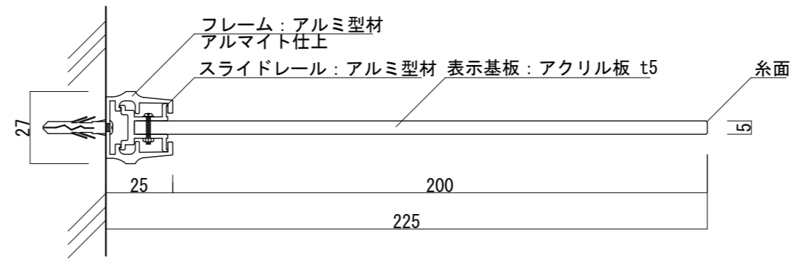
【平面図 S=1:2】
