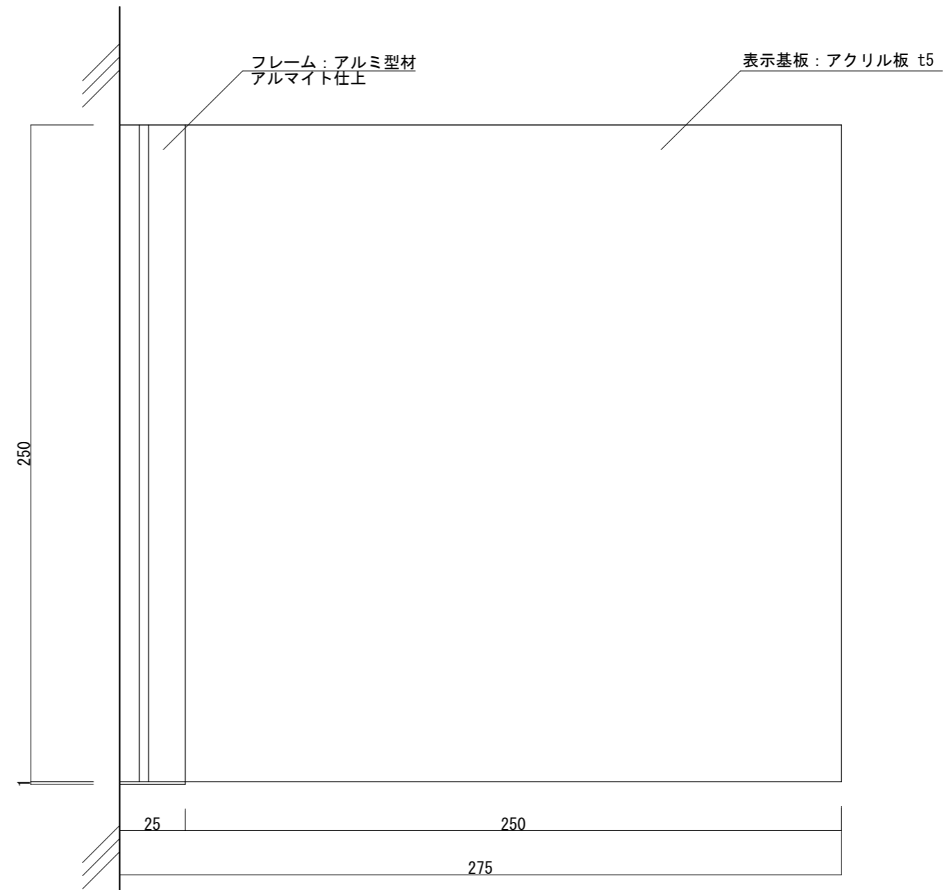
【正面図 S=1:2】
