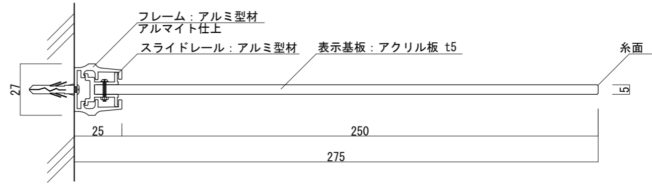
【平面図 S=1:2】
