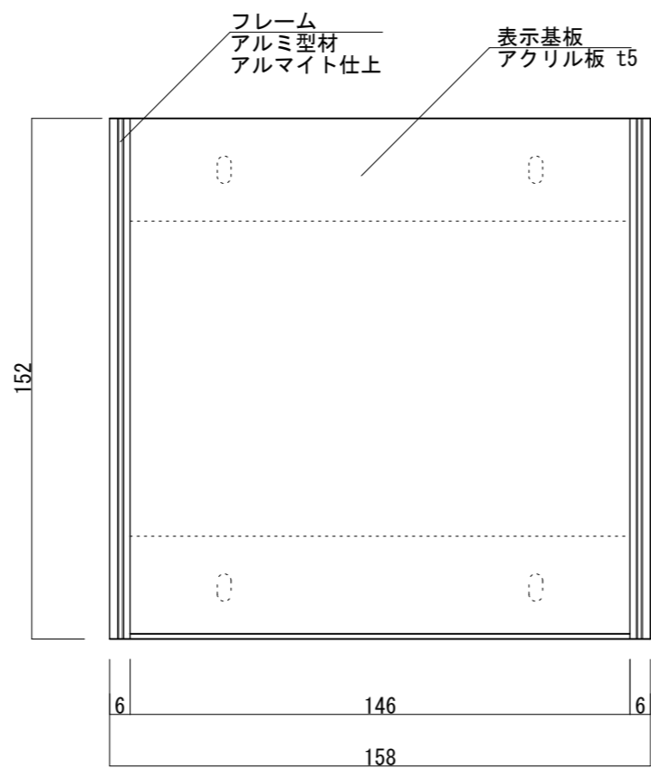
【正面図 S=1:2】
