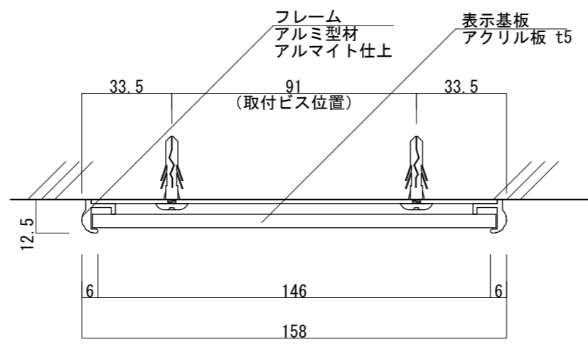
【平面図 S=1:2】
