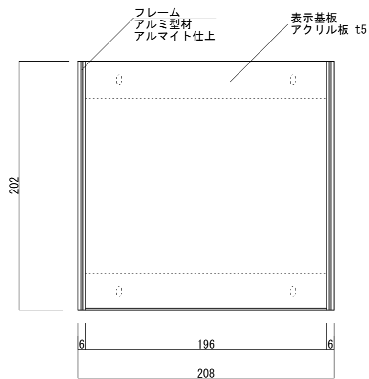
【正面図 S=1:3】
