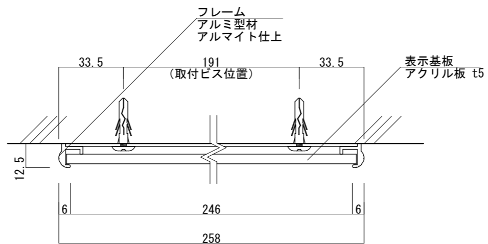
【平面図 S=1:2】
