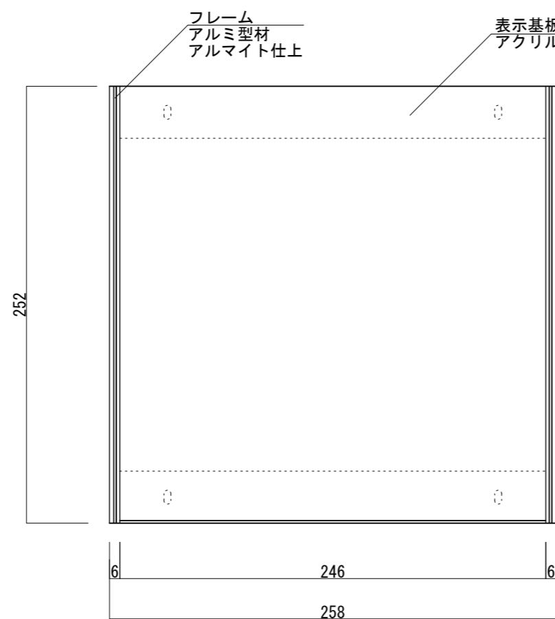
【正面図 S=1:3】
