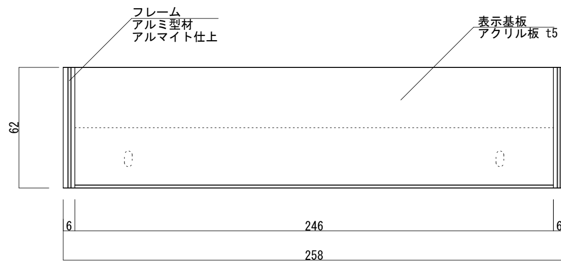
【正面図 S=1:2】
