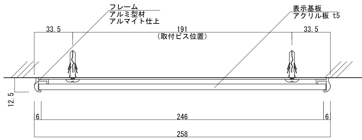
【平面図 S=1:2】
