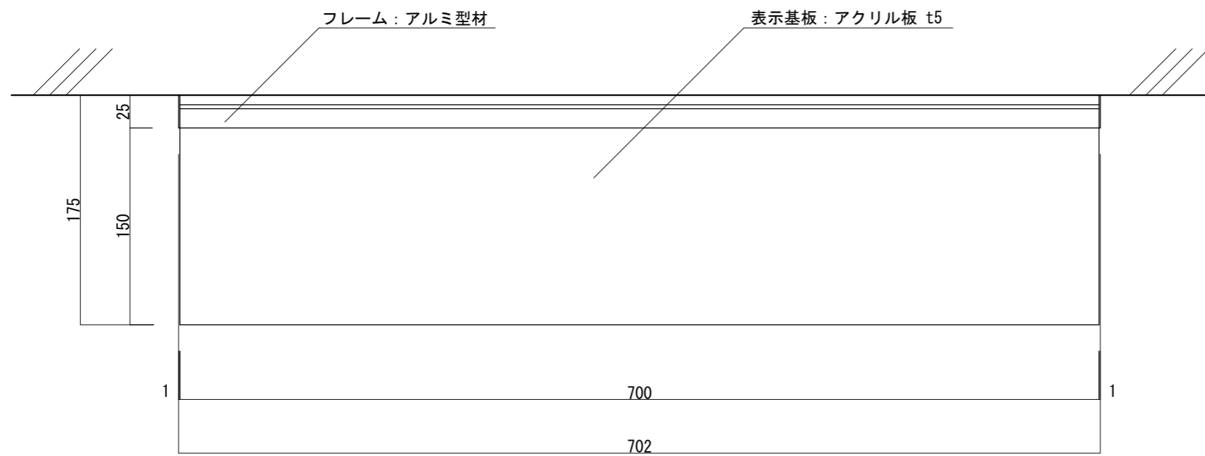
【正面図 S=1:4】
