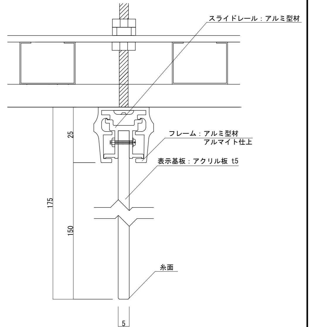
【断面図 S=1:1】
