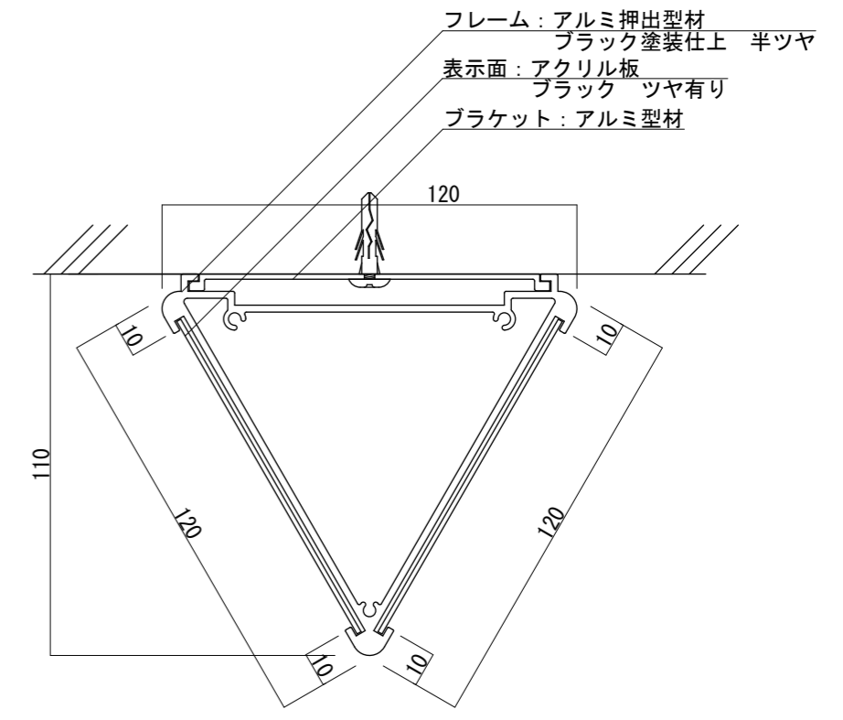
【断面図 S=1:2】
