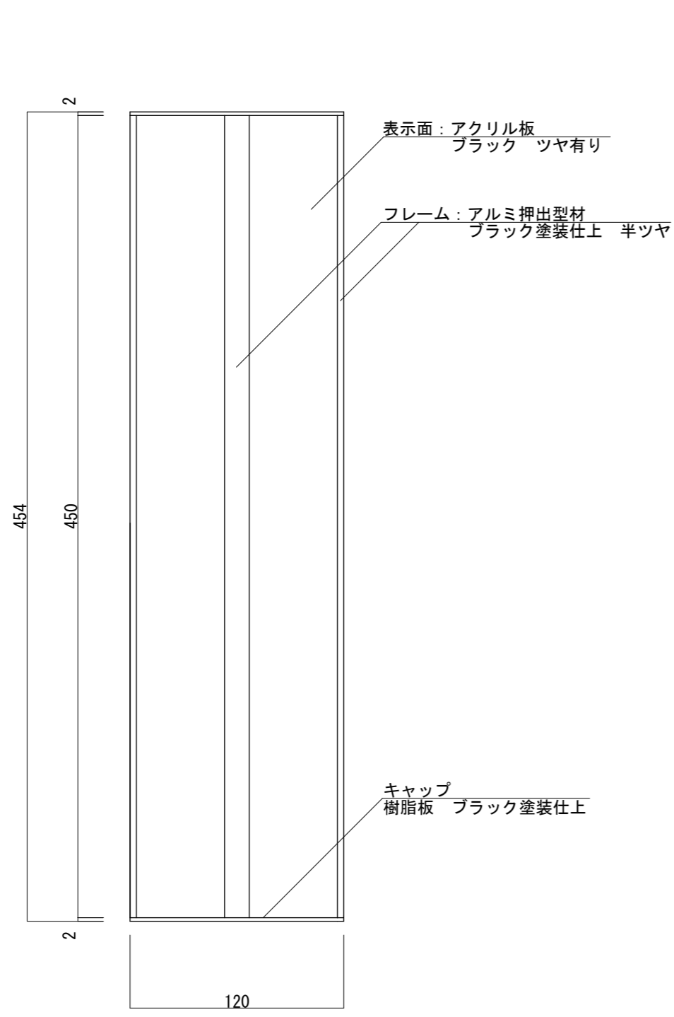
【正面図 S=1:3】
