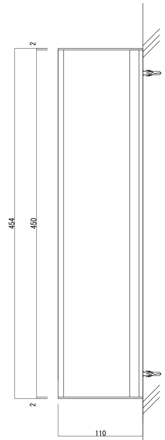
【側面図 S=1:3】
