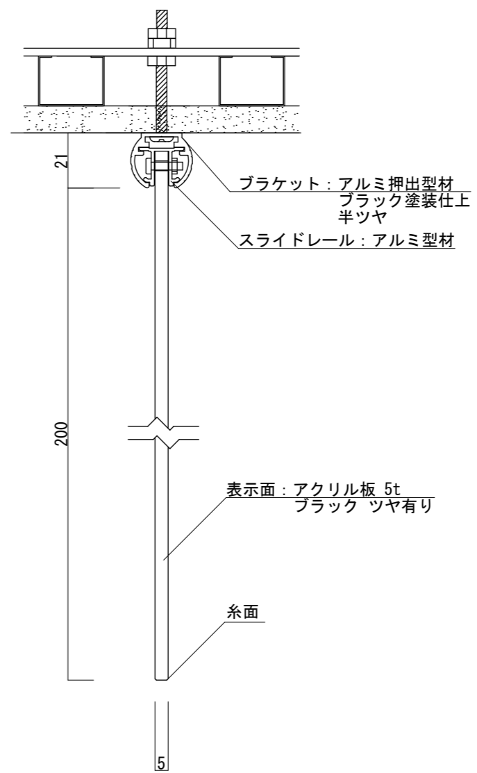
【断面図 S=1:2】
