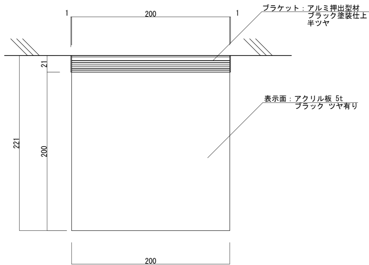
【正面図 S=1:3】
