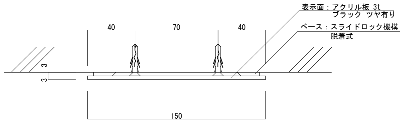
【平面図 S=1:2】
