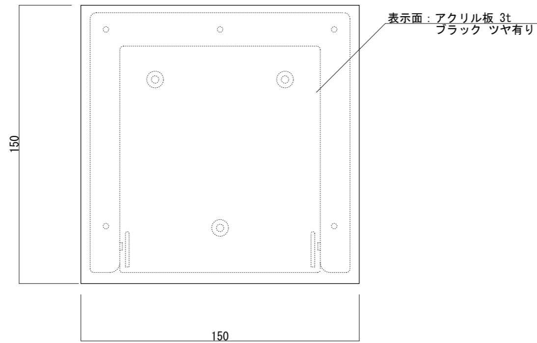
【正面図 S=1:2】
