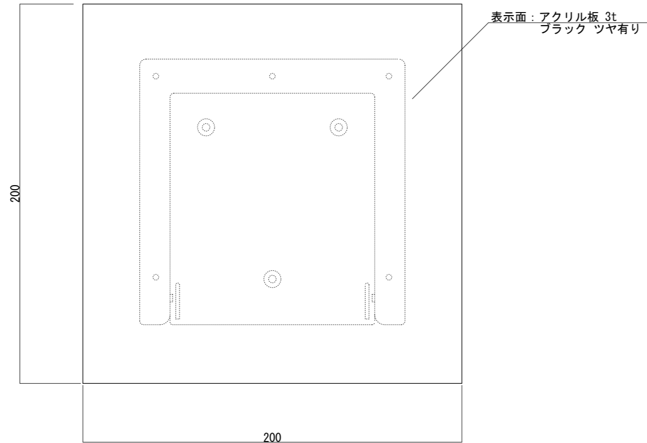
【正面図 S=1:2】
