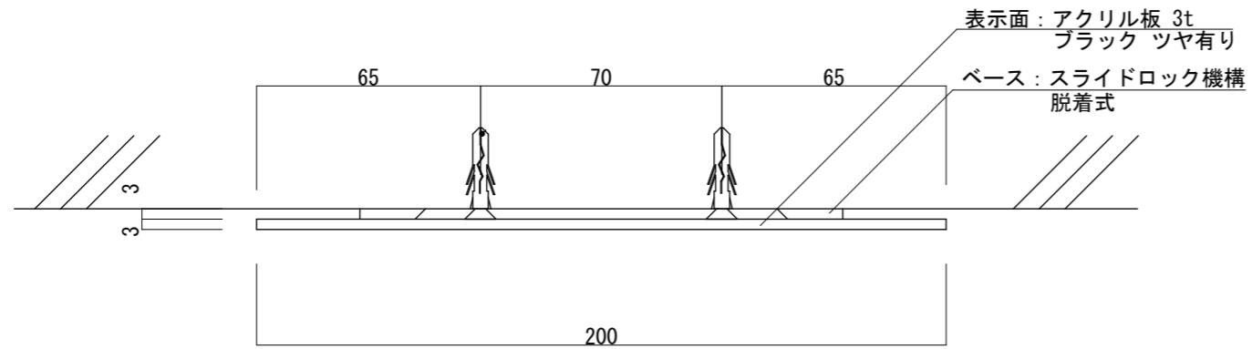
【平面図 S=1:2】
