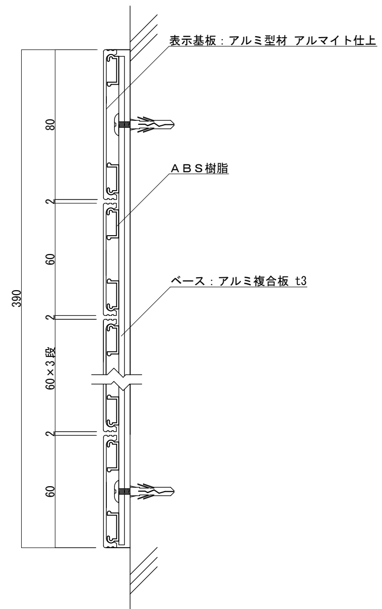
【側面図 S=1:2】
