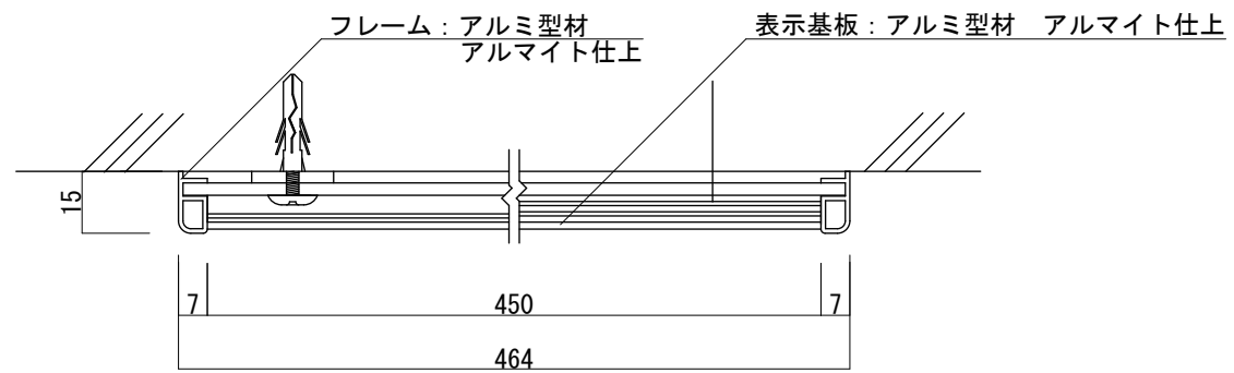
【平面図 S=1:2】
