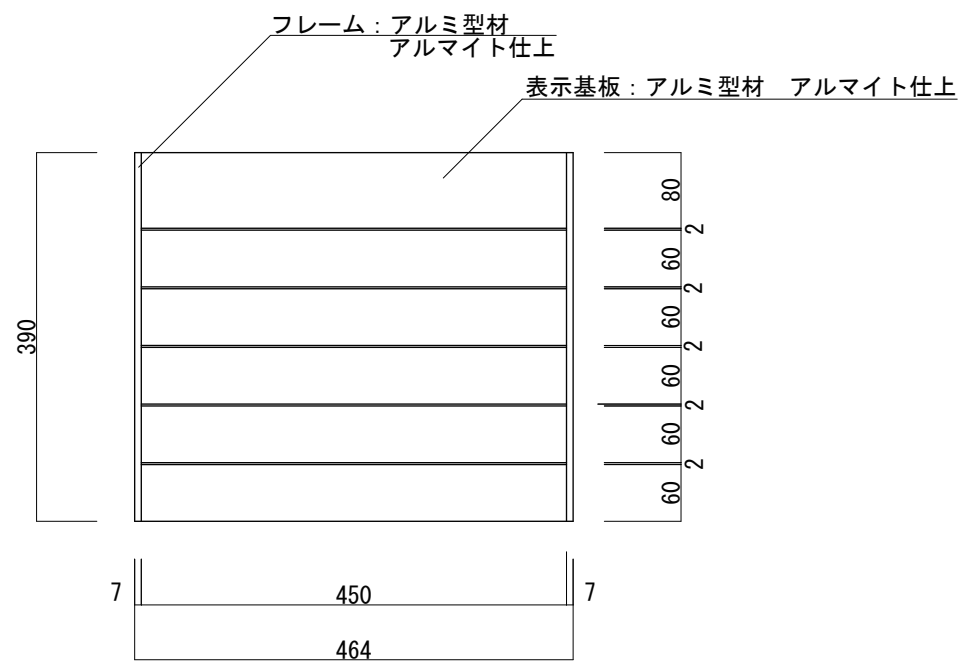
【正面図 S=1:8】
