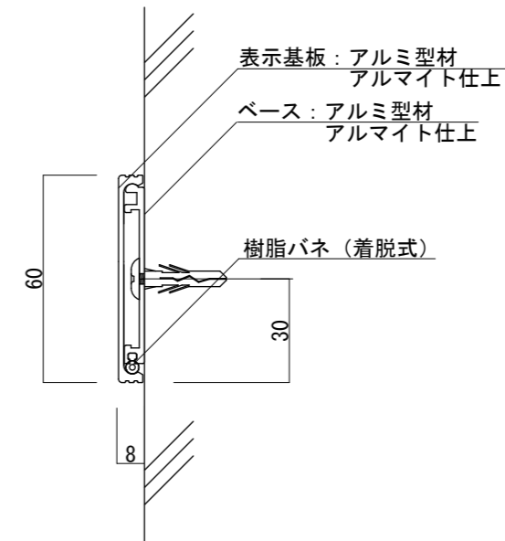
【側面図 S=1:2】
