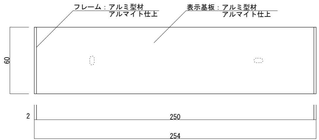
【正面図 S=1:2】
