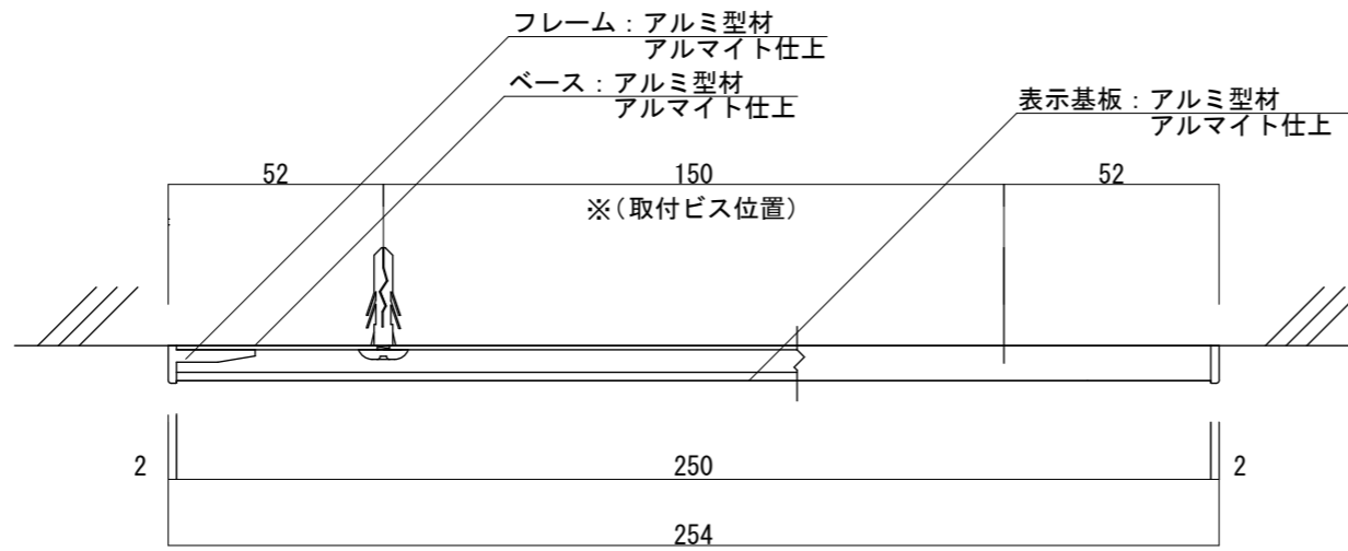
【平面図 S=1:2】
