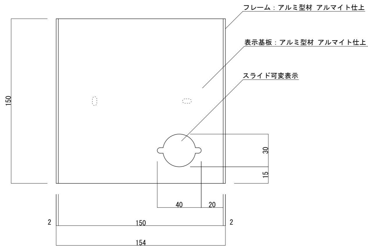
【正面図 S=1:2】
