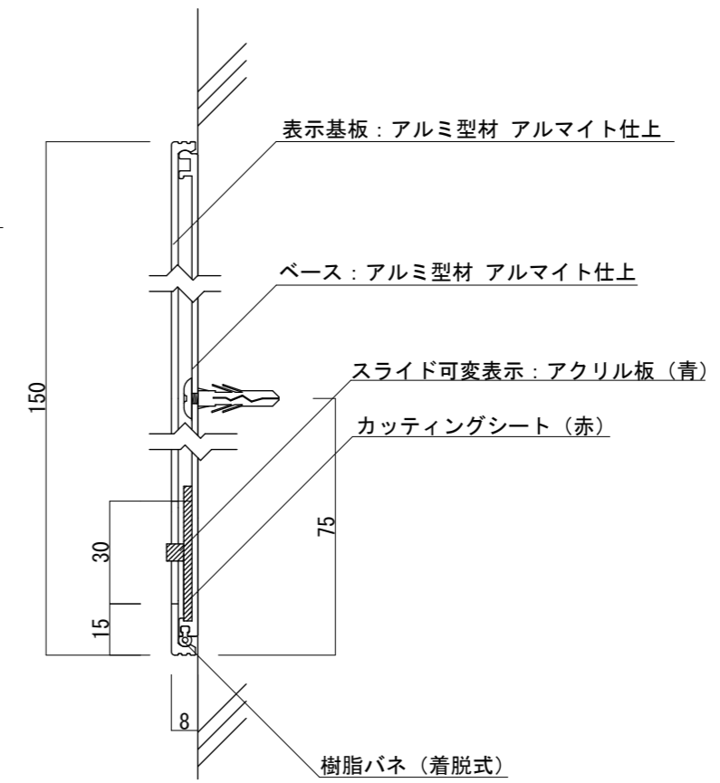
【側面図 S=1:2】
