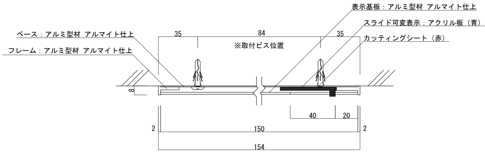
【平面図 S=1:2】
