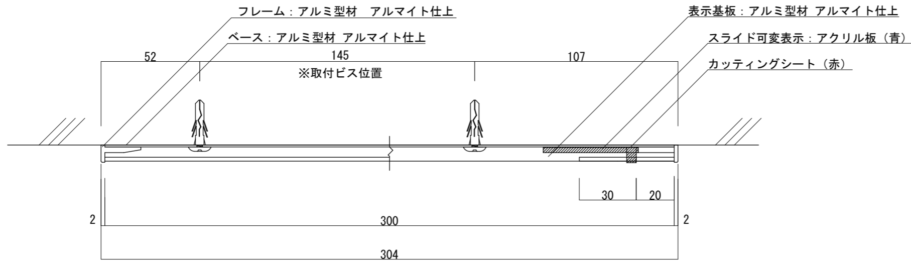
【平面図 S=1:2】
