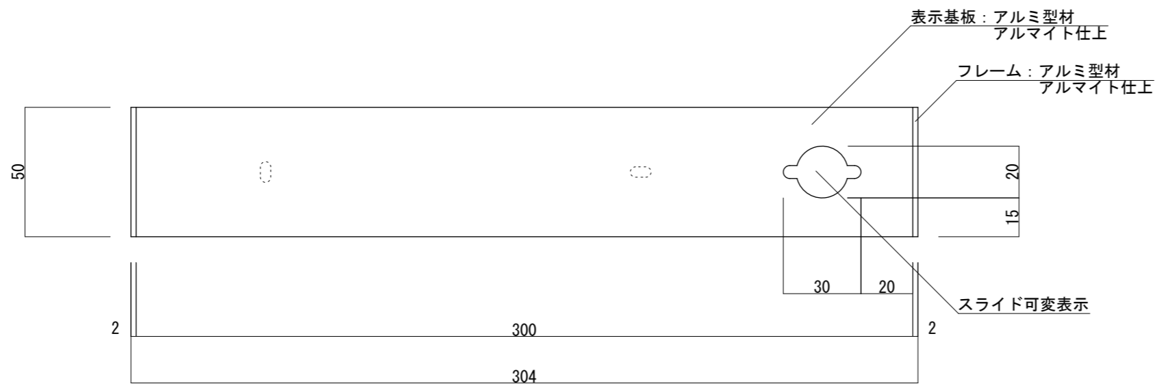
【正面図 S=1:2】
