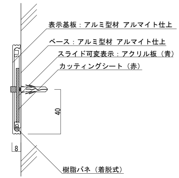
【側面図 S=1:2】
