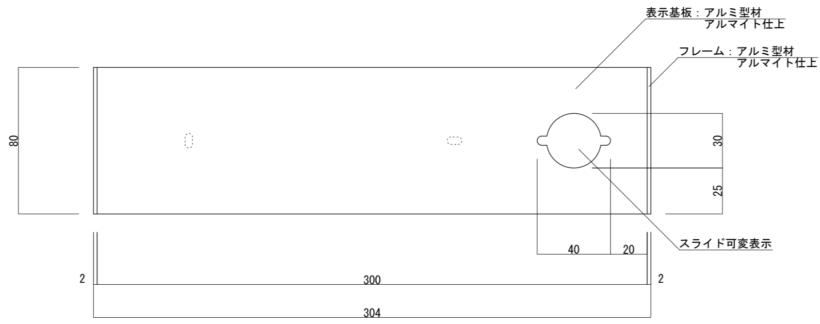
【正面図 S=1:2】
