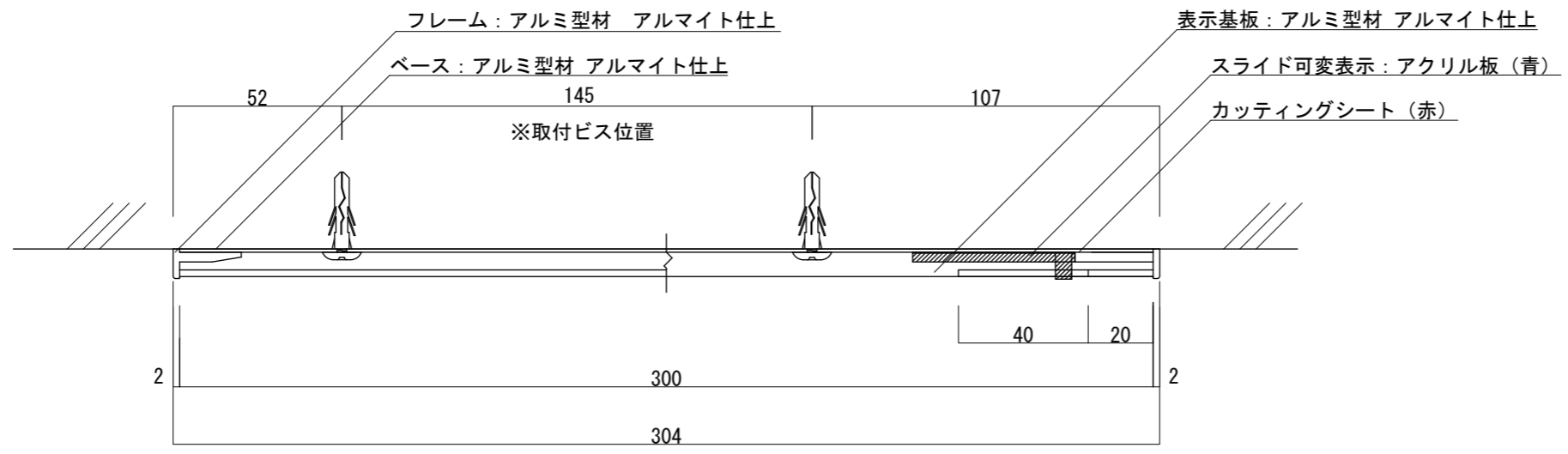
【平面図 S=1:2】
