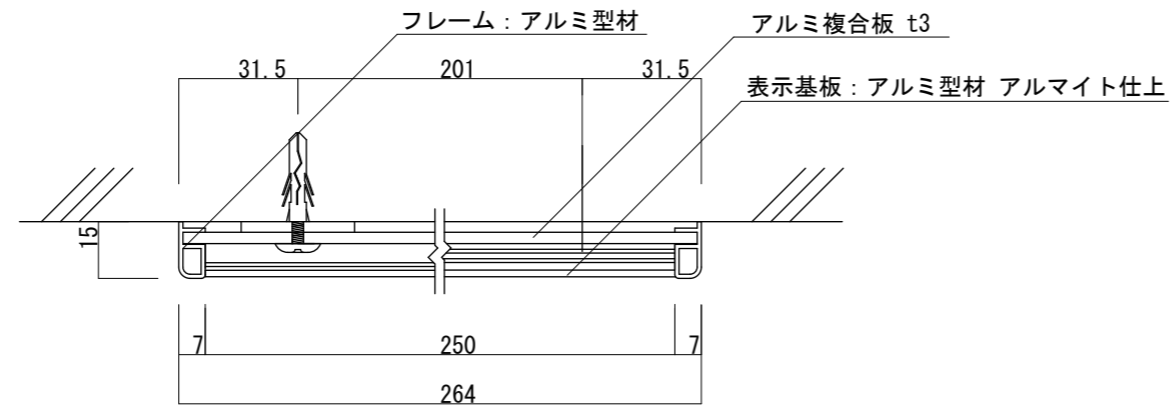
【断面図 S=1:2】
