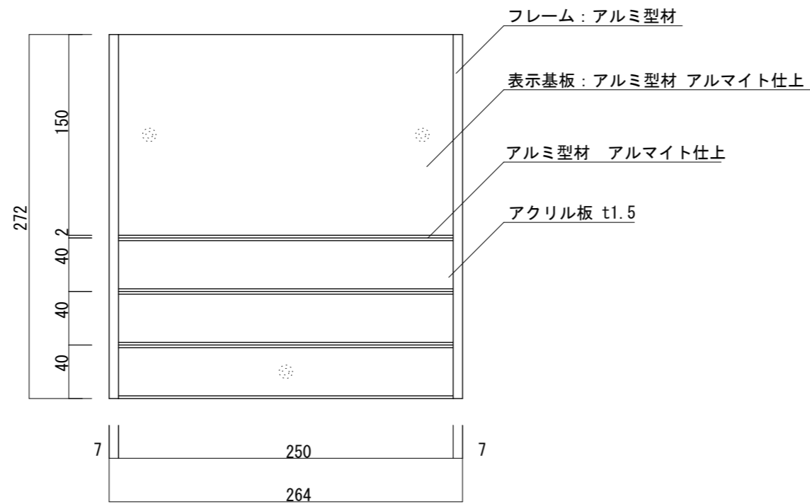
【正面図 S=1:4】
