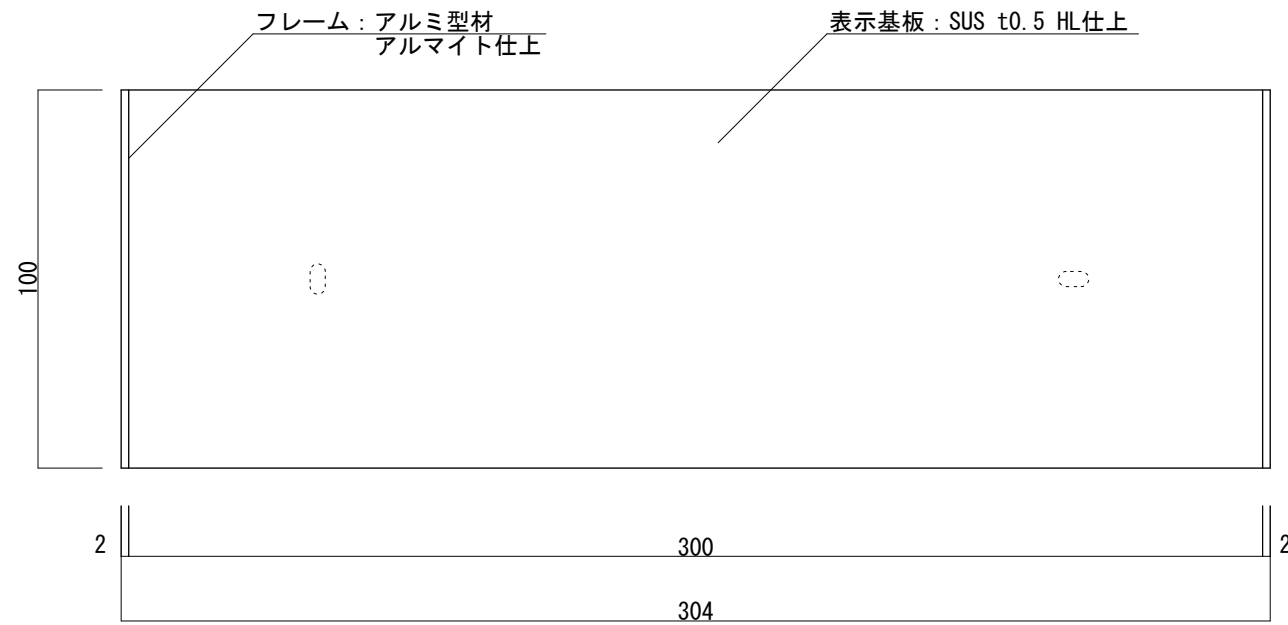
【正面図 S=1:2】
