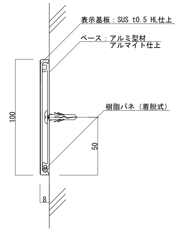
【側面図 S=1:2】
