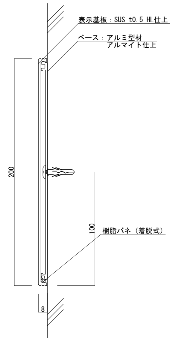
【側面図 S=1:2】
