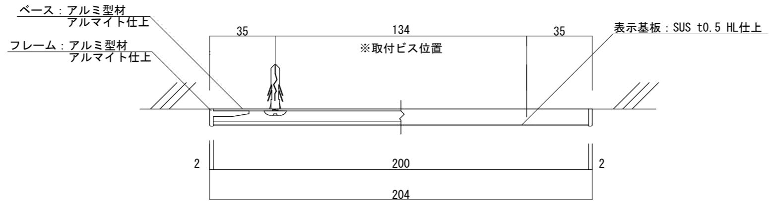
【平面図 S=1:2】
