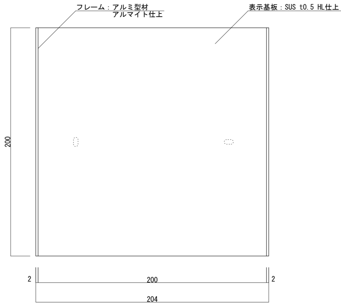
【正面図 S=1:2】
