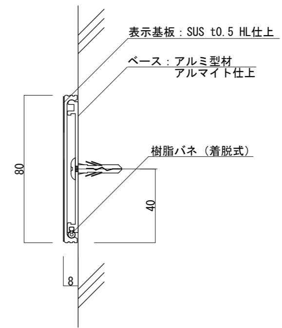
【側面図 S=1:2】
