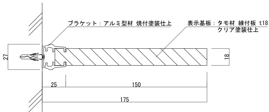
【平面図 S=1:2】
