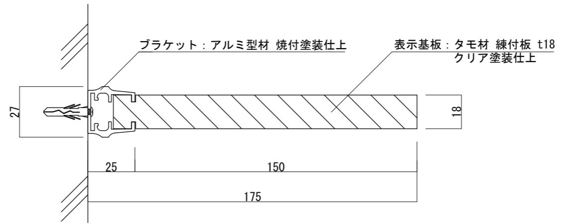
【平面図 S=1:2】
