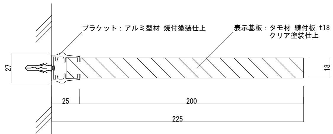
【平面図 S=1:2】
