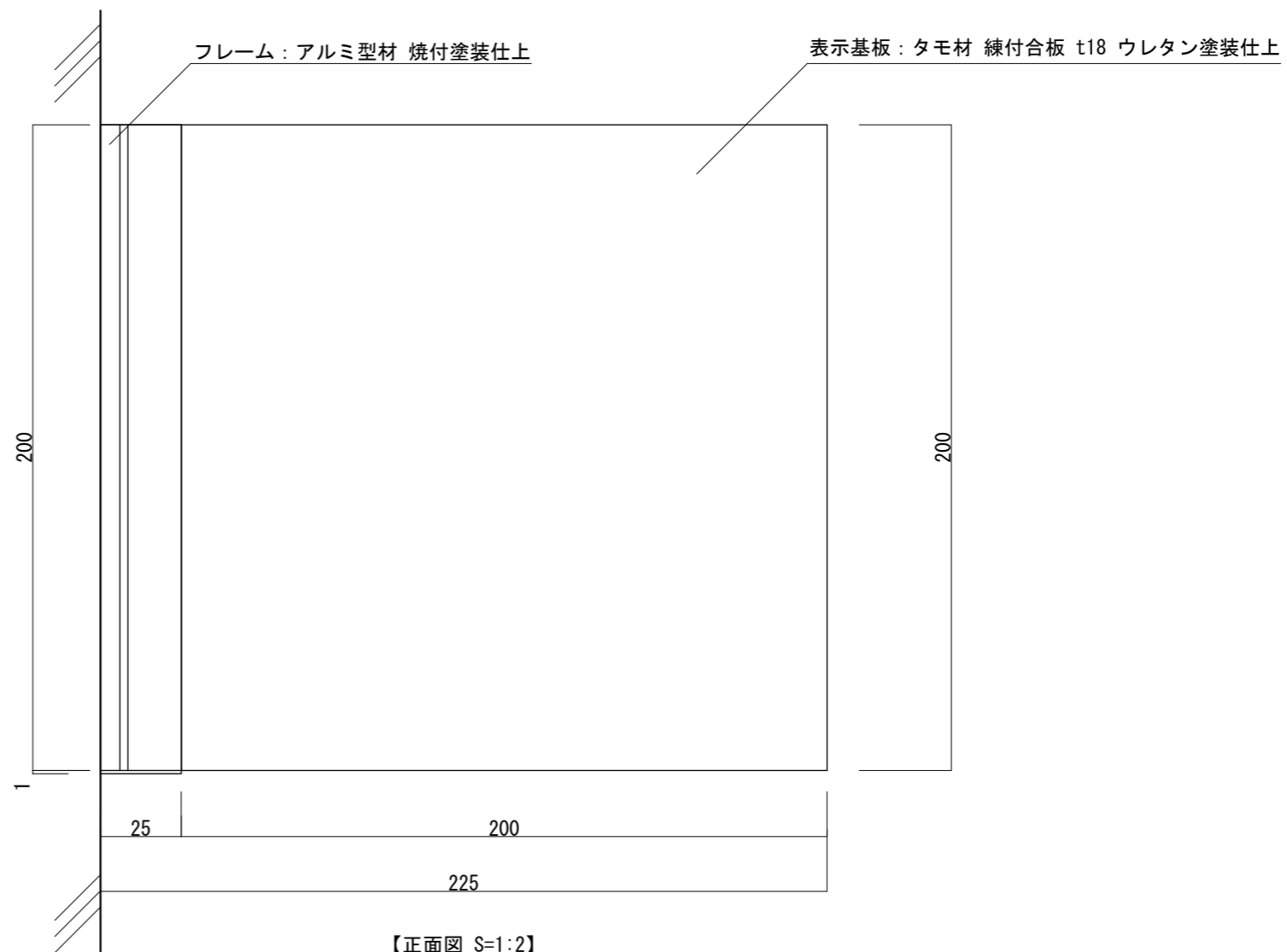
【正面図 S=1:2】
