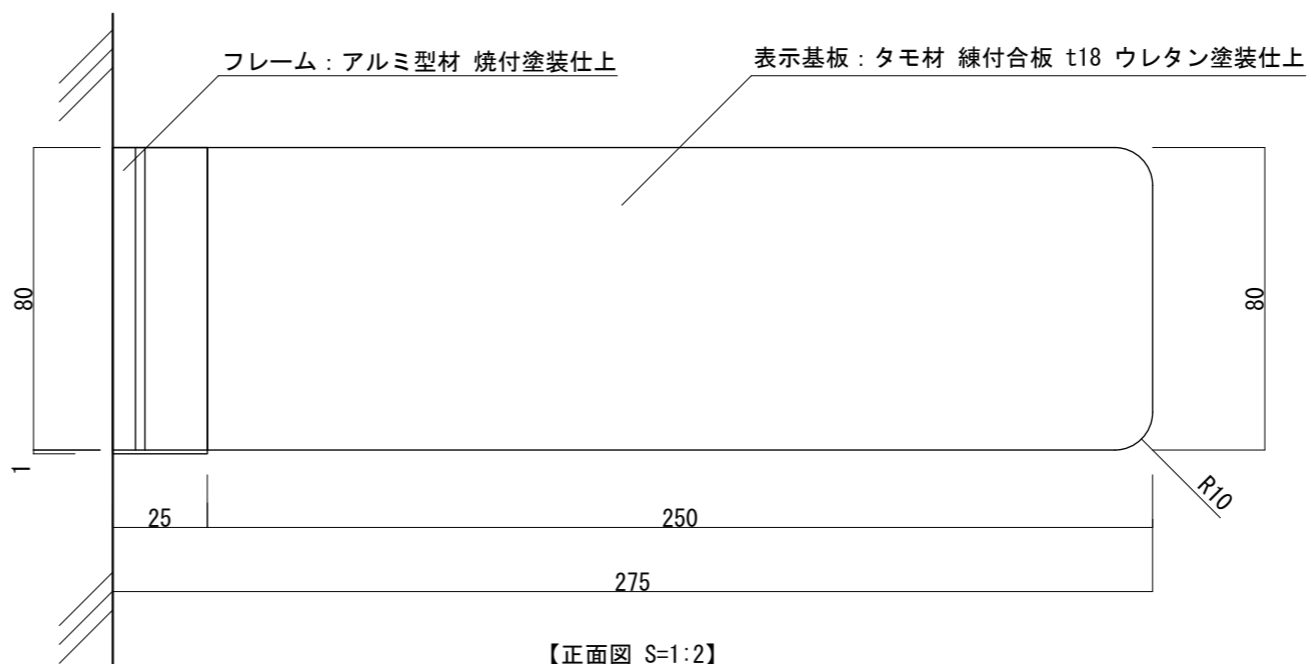
【正面図 S=1:2】
