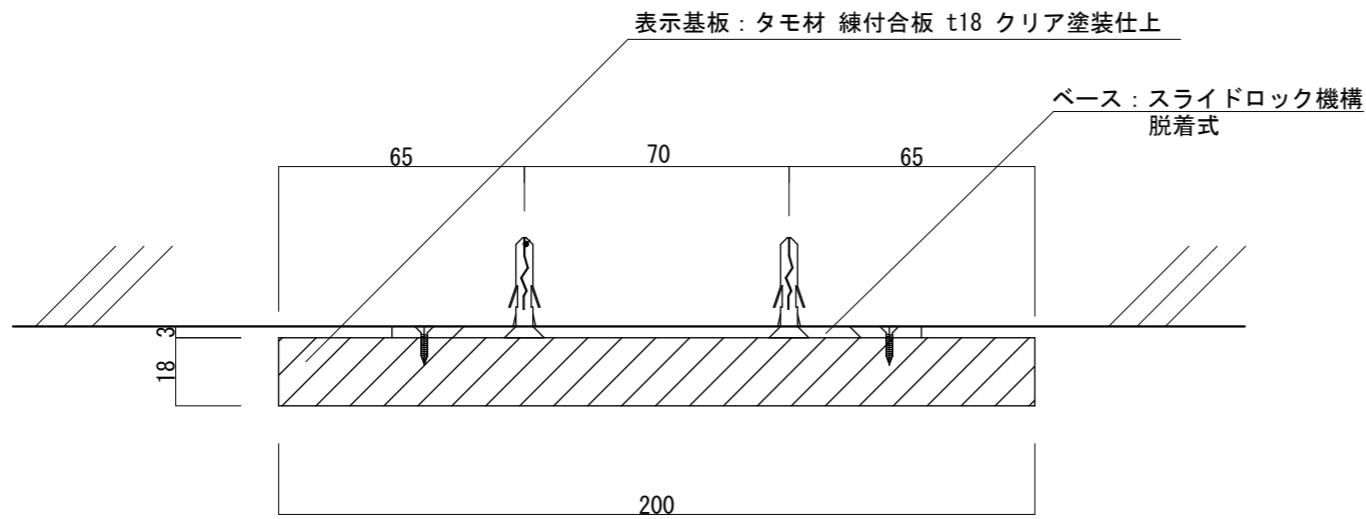
【平面図 S=1:2】
