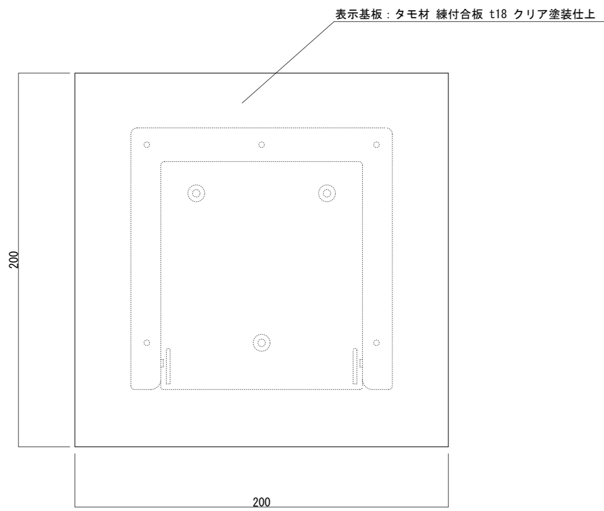
【正面図 S=1:2】
