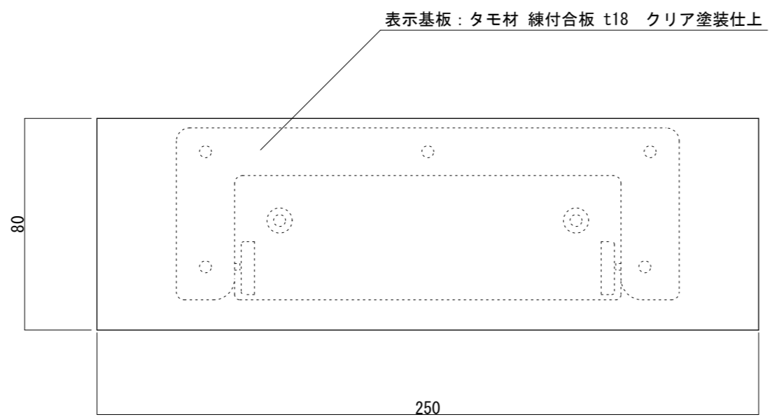
【正面図 S=1:2】
