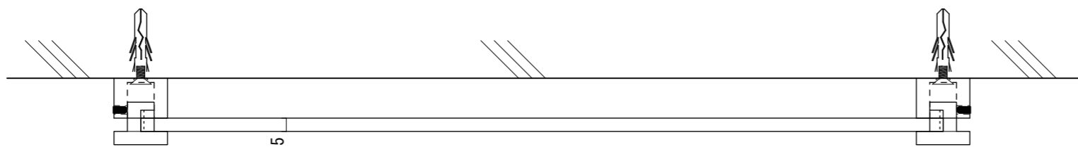
【平面図 S=1:2】
