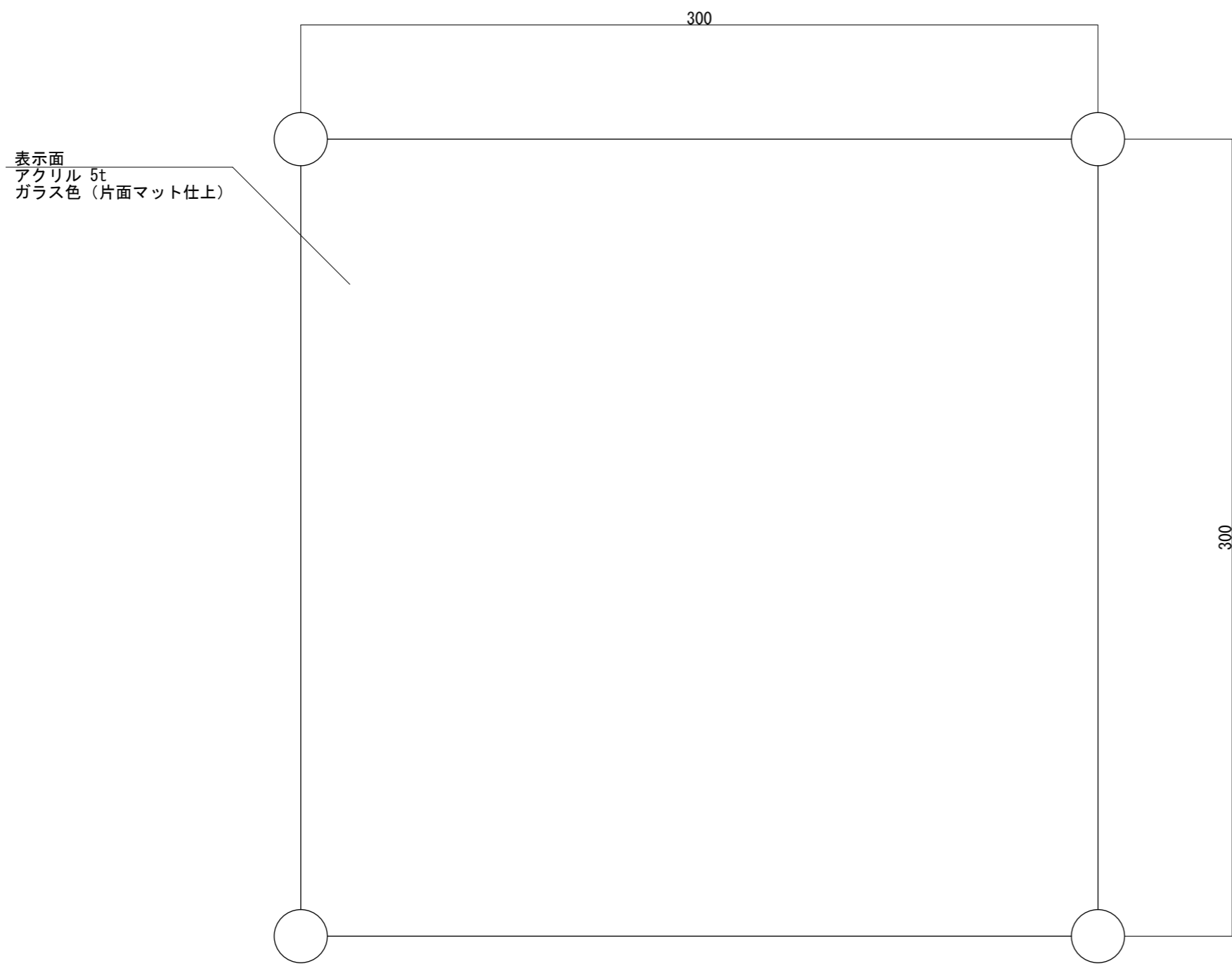
【正面図 S=1:2】
