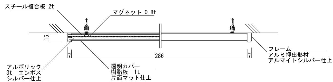
【詳細図 S=1:3】
