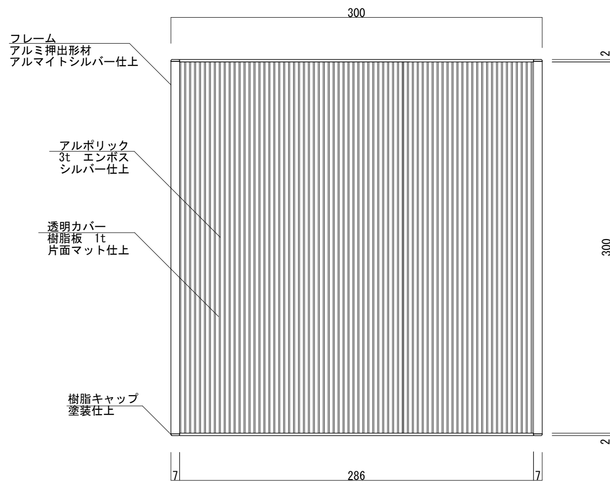
【正面図 S=1:3】
