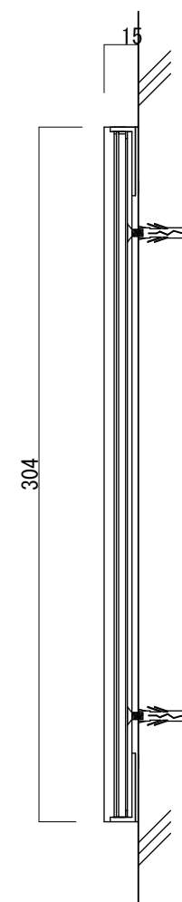
【側断面図 S=1:3】
