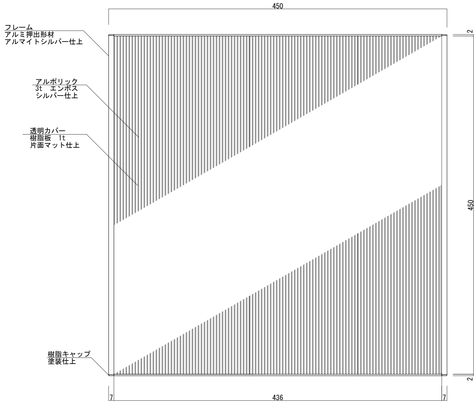
【正面図 S=1:3】
