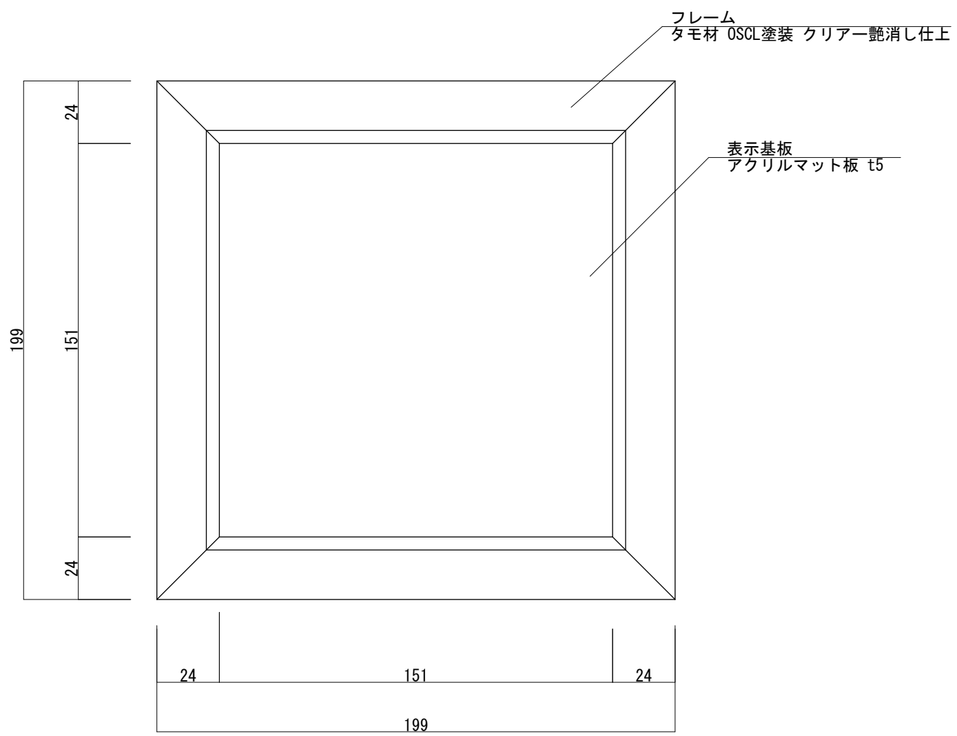
【正面図 S=1:2】
