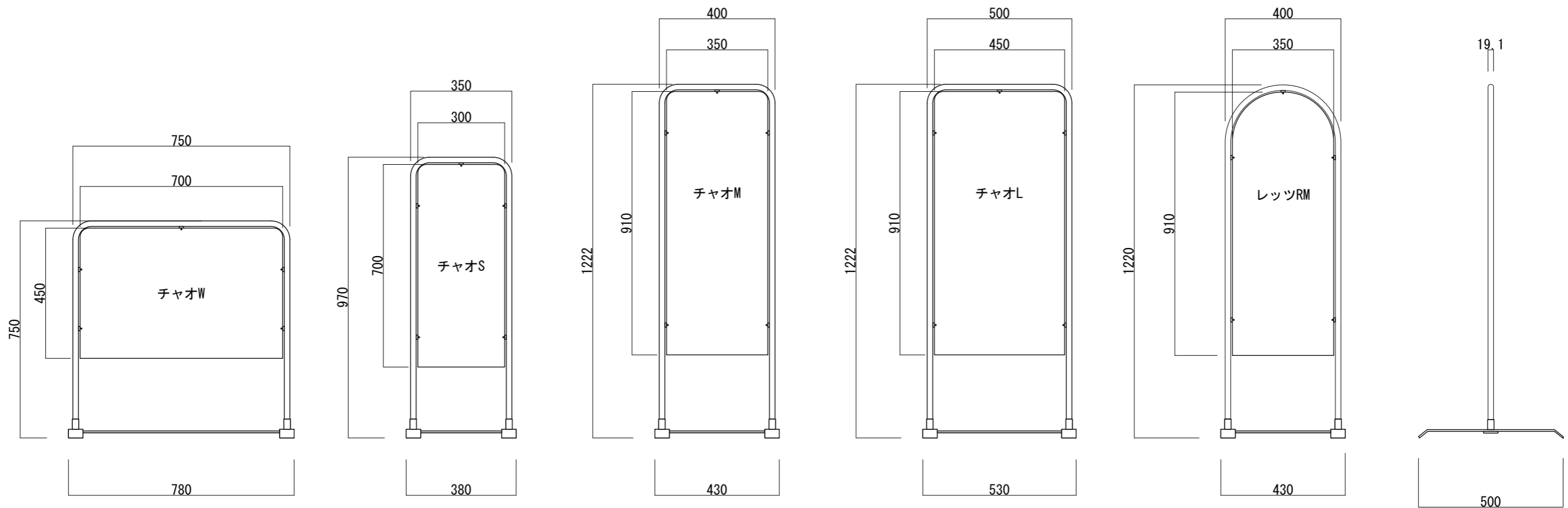
【正面図 S=1:15】
