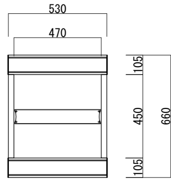
【平面図 S=1:20】
