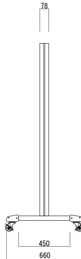
【側面図 S=1:20】
