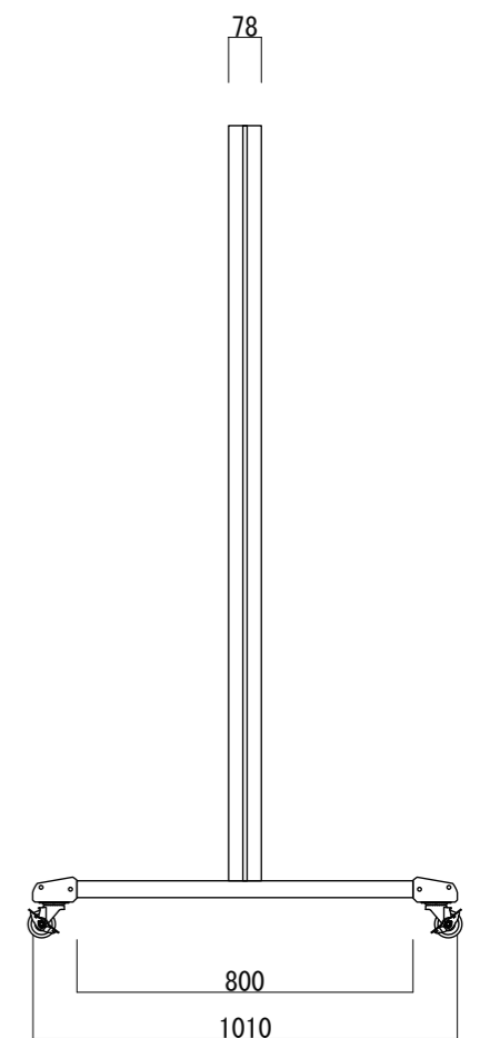
【側面図 S=1:20】
