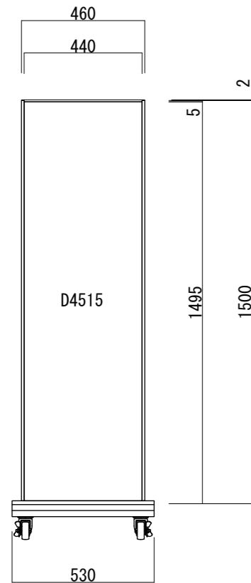
【正面図 S=1:20】
