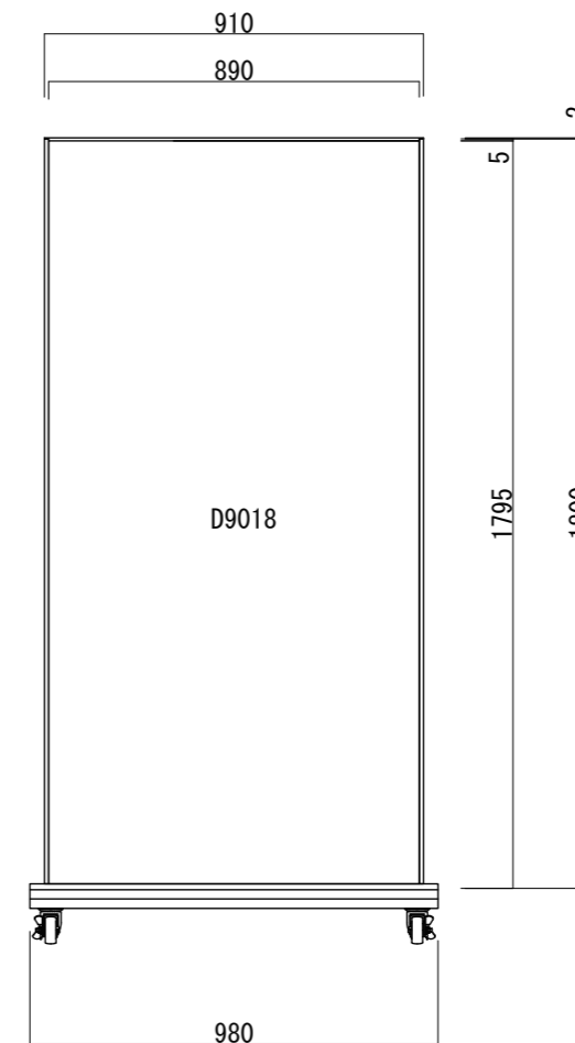
【正面図 S=1:20】
