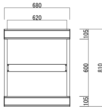
【平面図 S=1:20】
