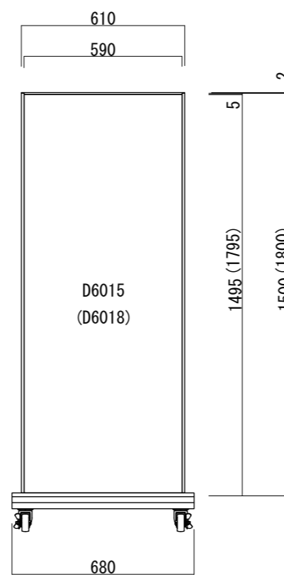
【正面図 S=1:20】
