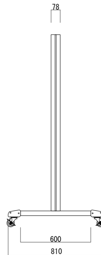
【側面図 S=1:20】
