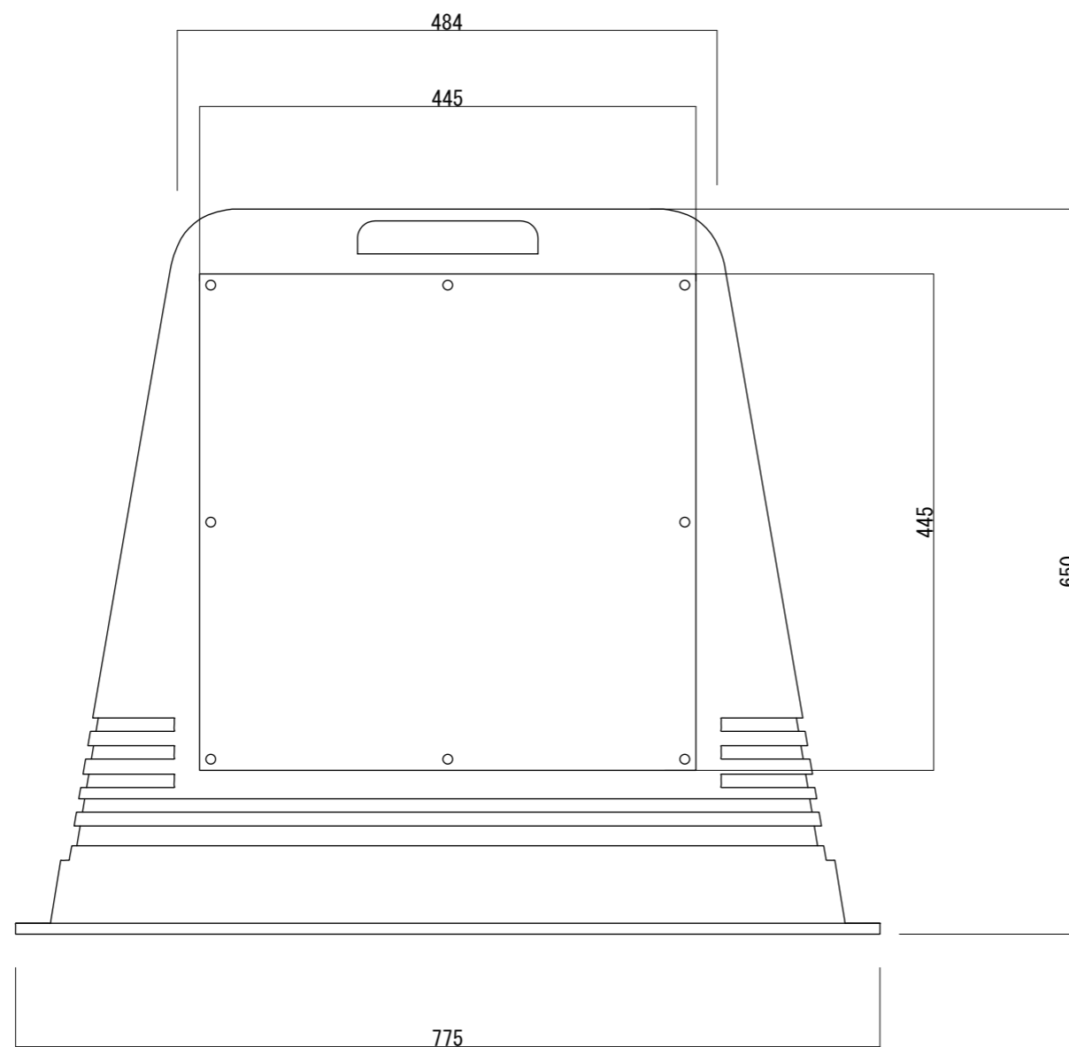
【正面図 S=1:6】
