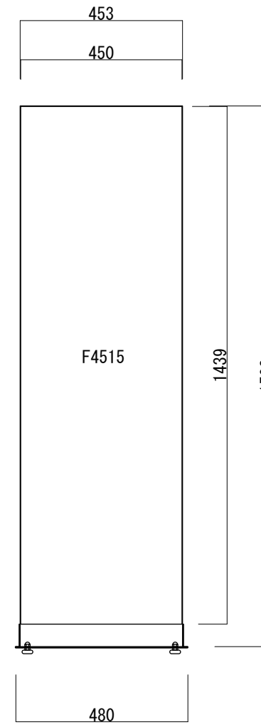
【正面図 S=1:15】
