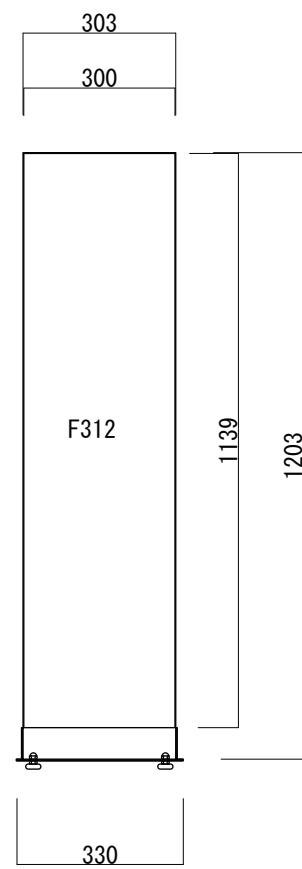
【正面図 S=1:15】
