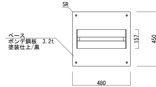
【平面図 S=1:15】
