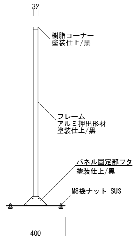
【側面図 S=1:15】
