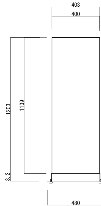
【正面図 S=1:15】
