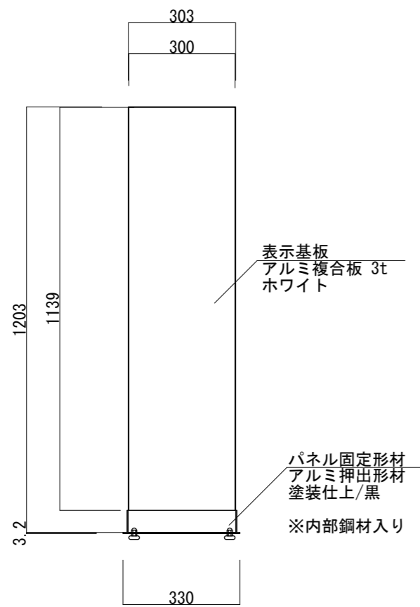
【正面図 S=1:15】
