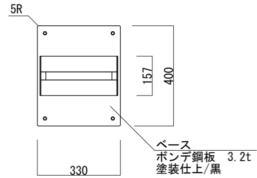
【平面図 S=1:15】
