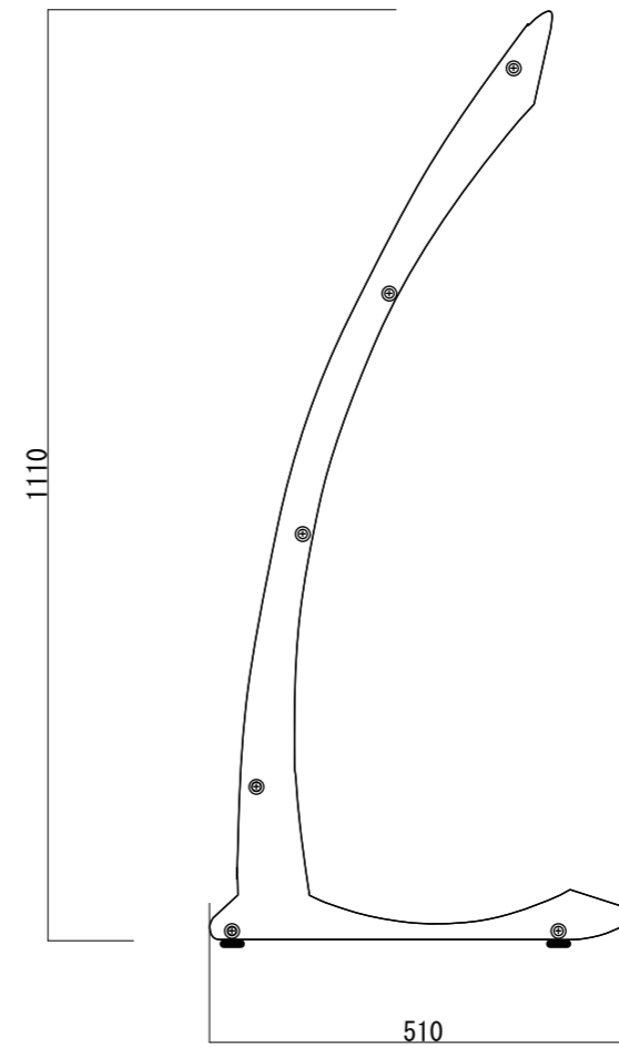
【側面図 S=1:10】
