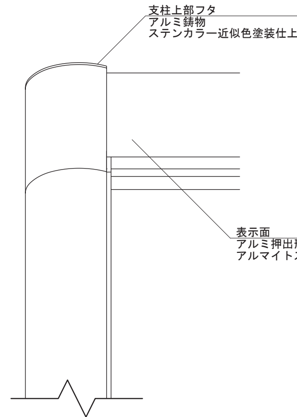
【正面図 S=1:5】
