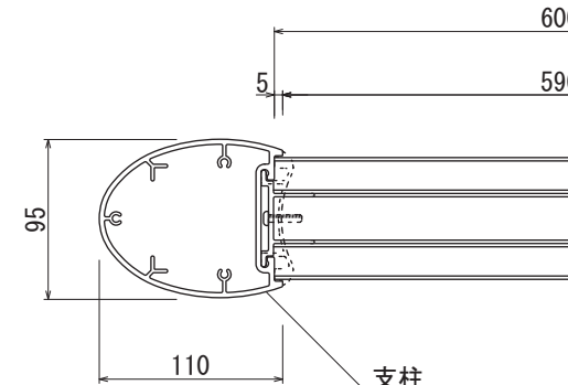
【平面図 S=1:5】
