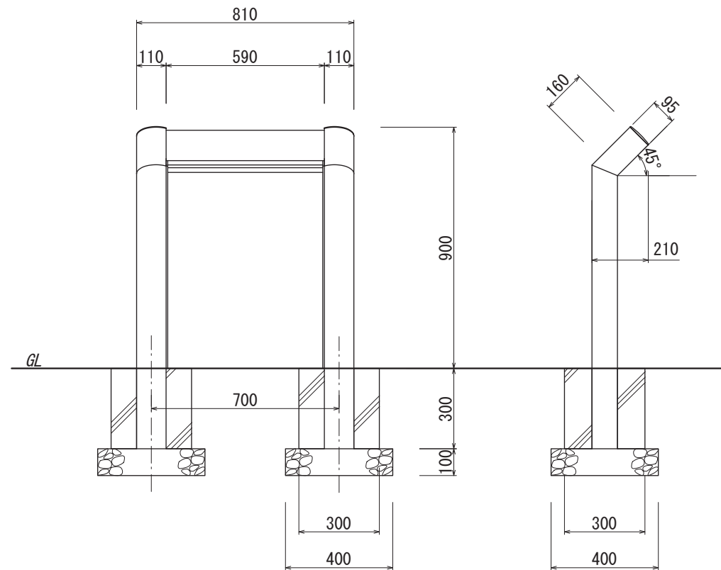
【正面図 S=1:20】
