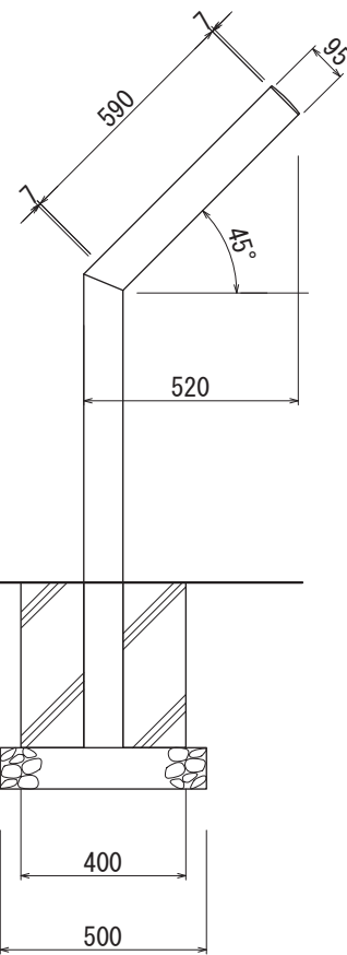
【側面図 S=1:20】
