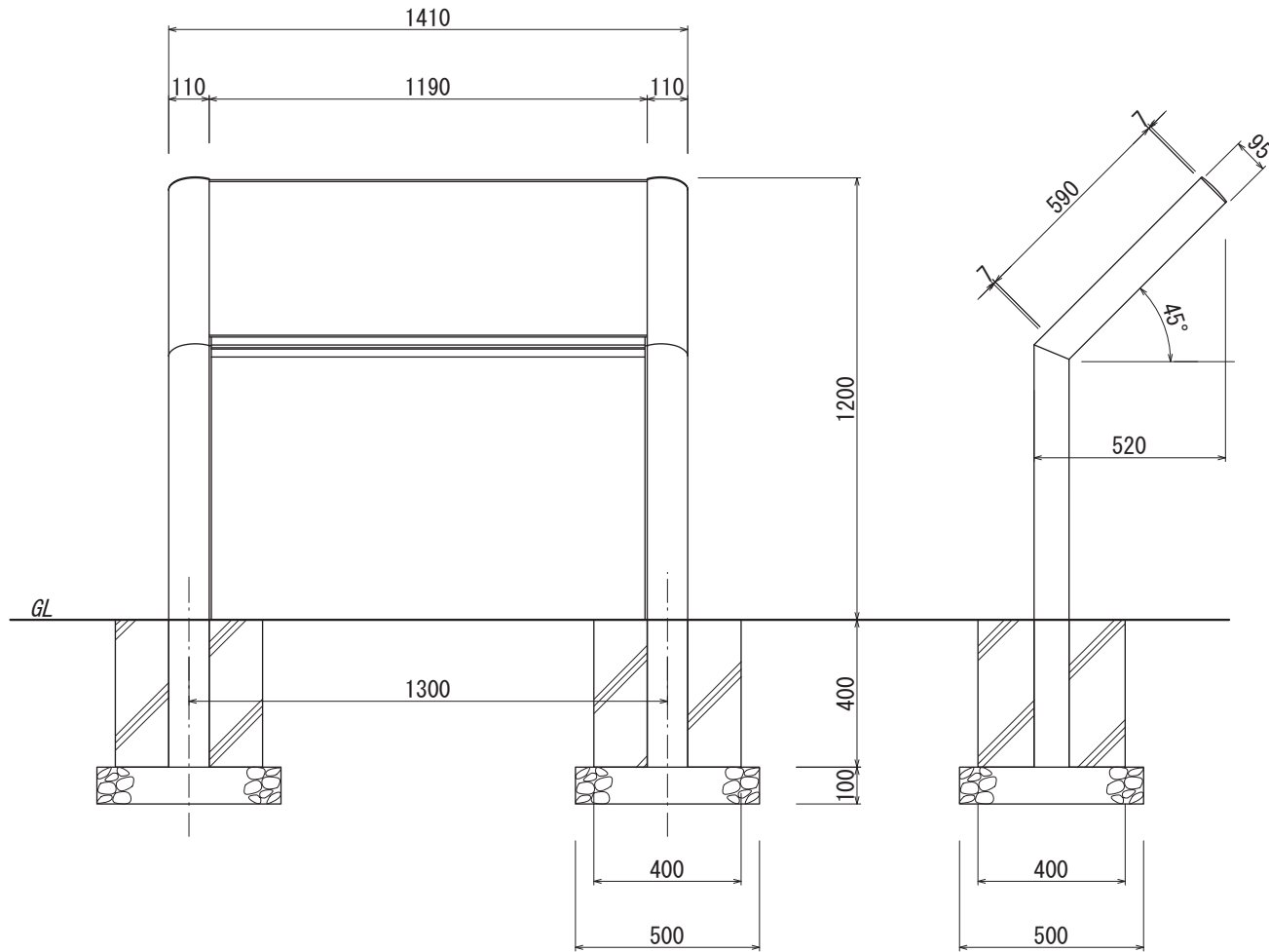
【正面図 S=1:20】
