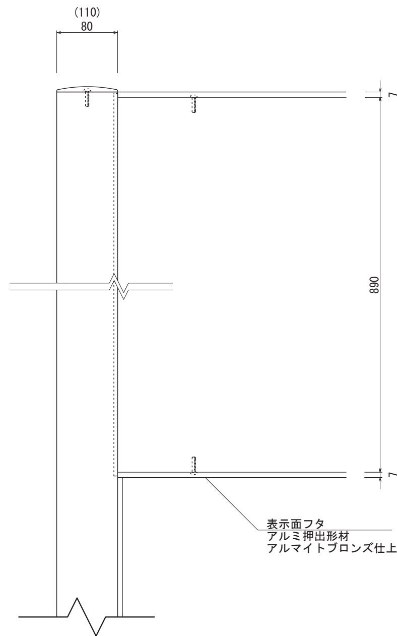
【正面図 S=1:5】
