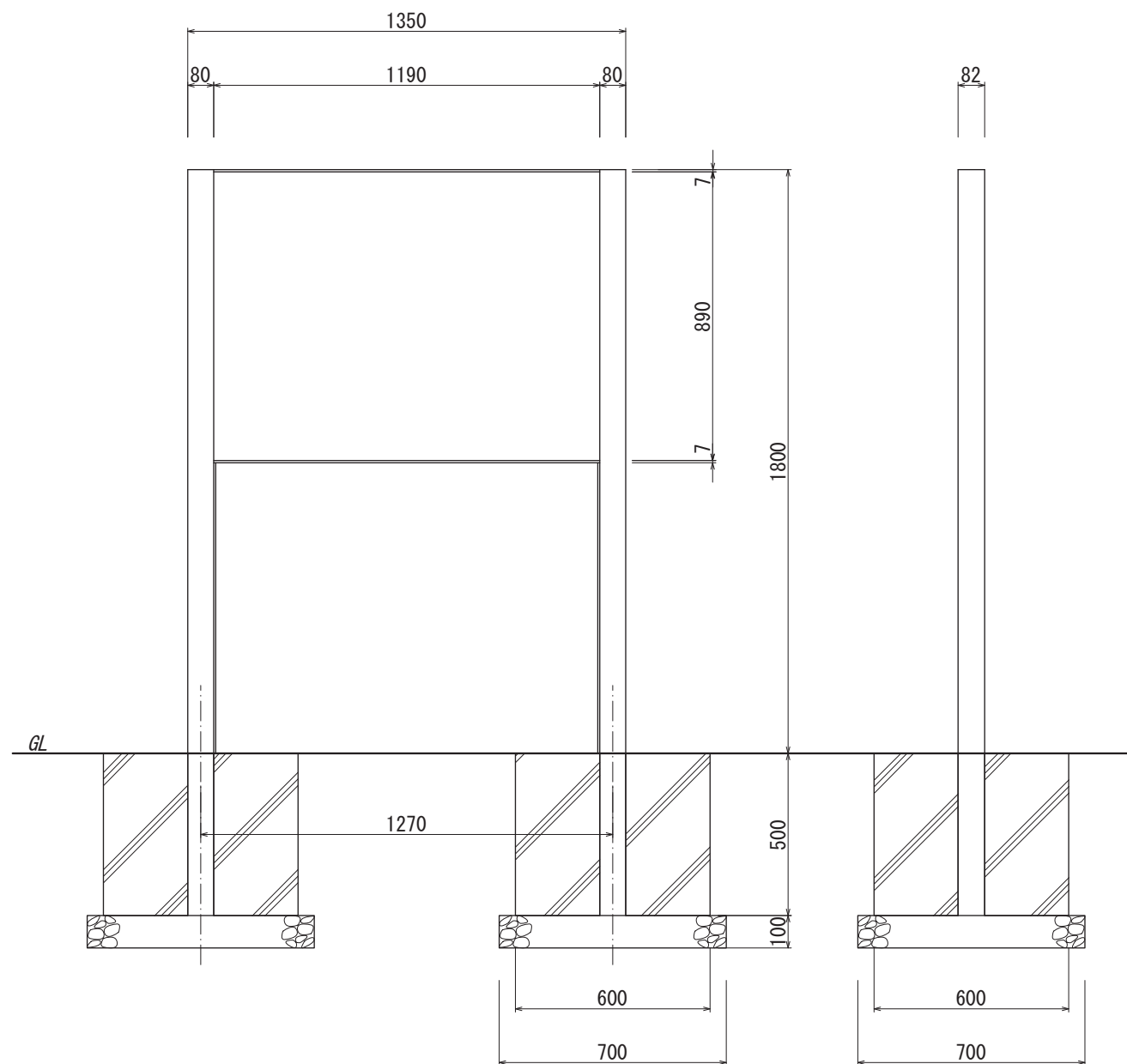
【正面図 S=1:20】
