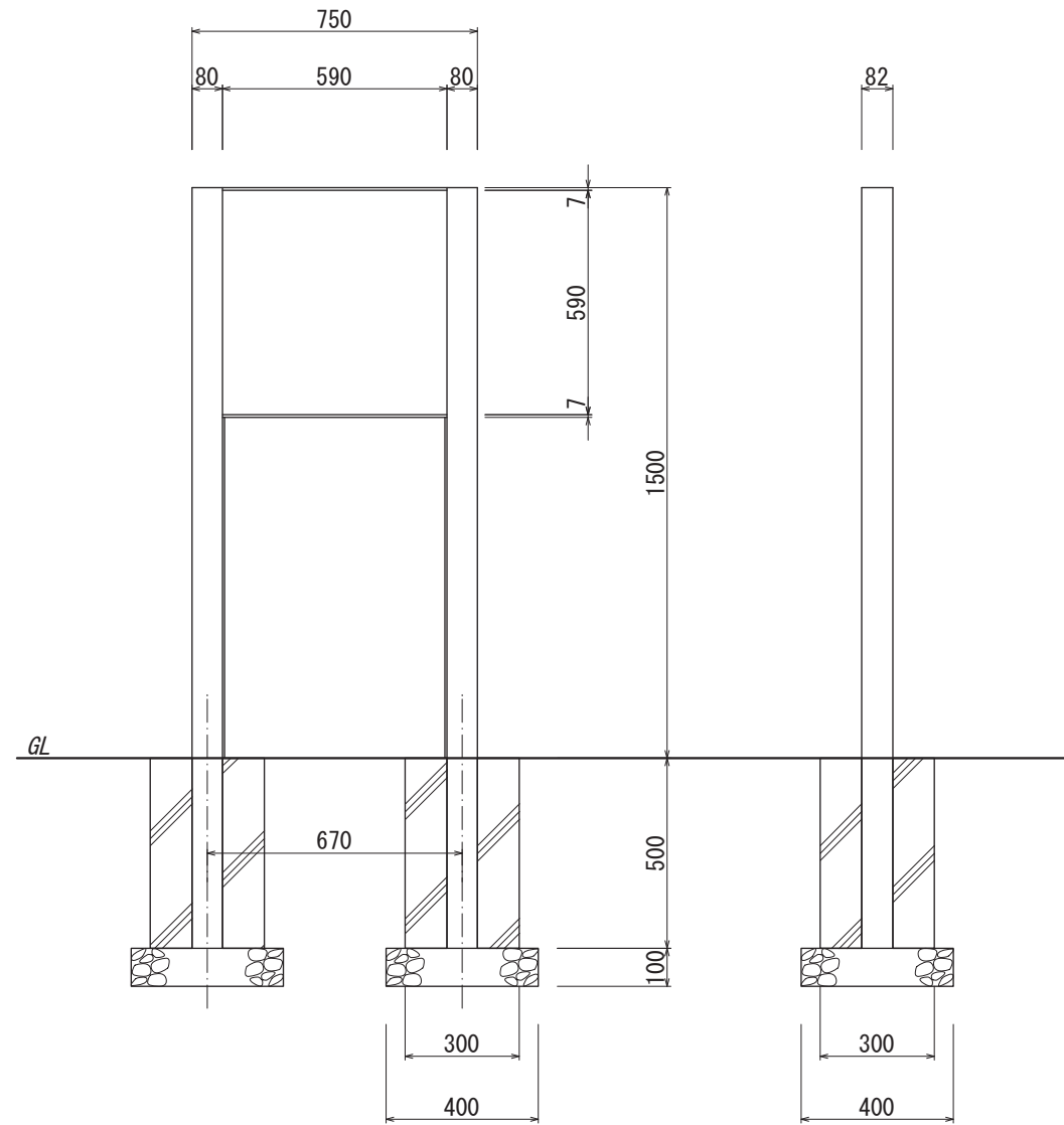
【正面図 S=1:20】
