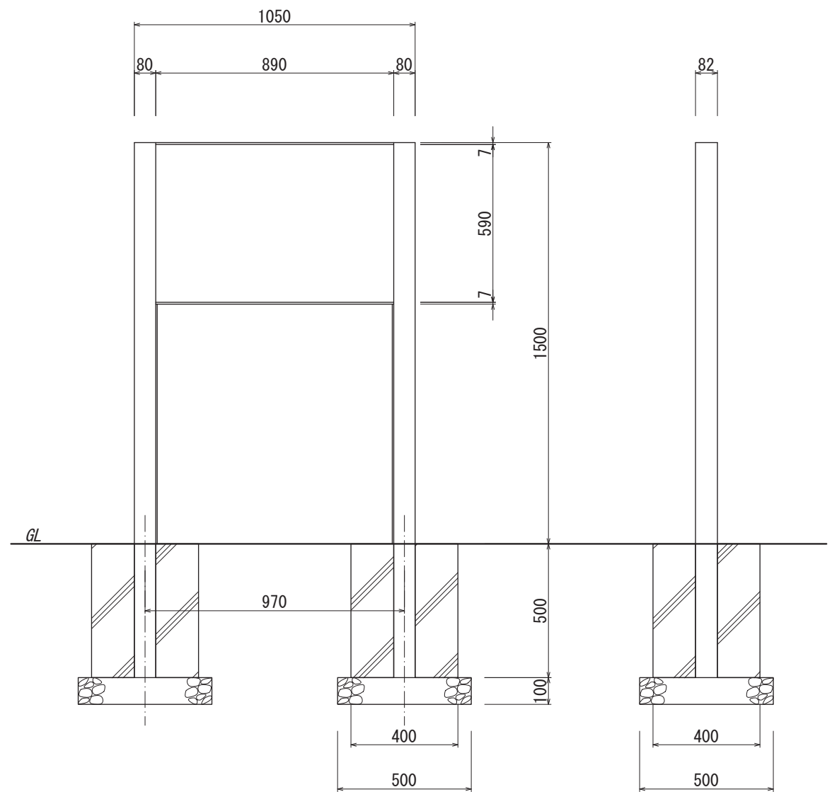
【正面図 S=1:20】
