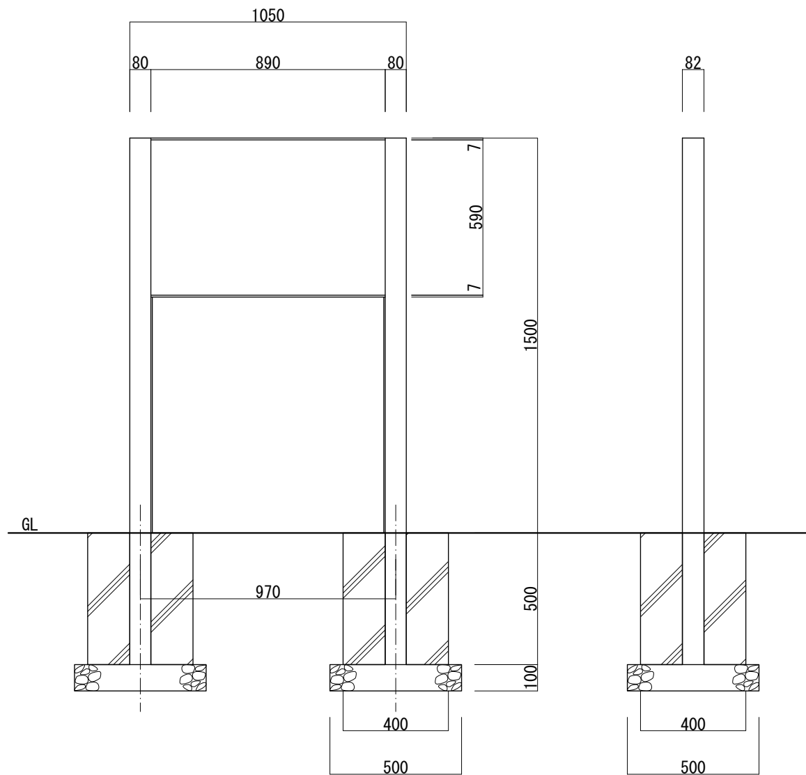
【側面図 S=1:20】
