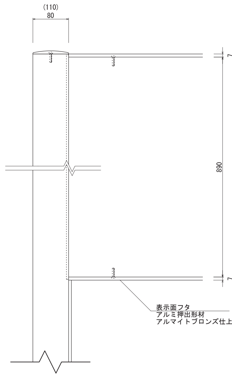
【正面図 S=1:5】
