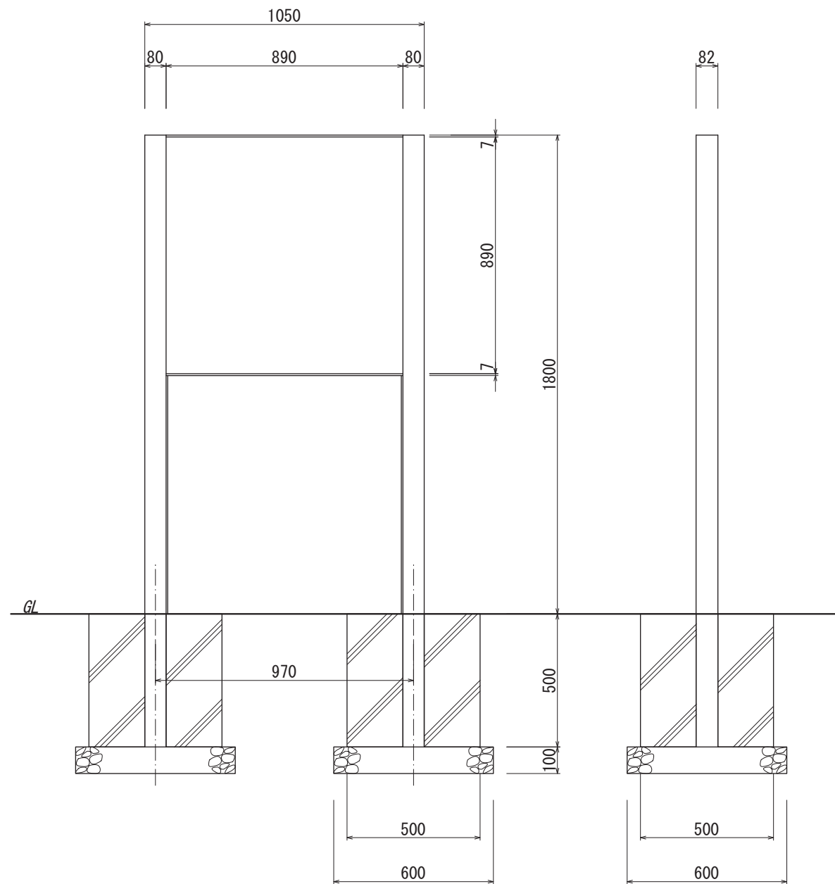
【正面図 S=1:20】
