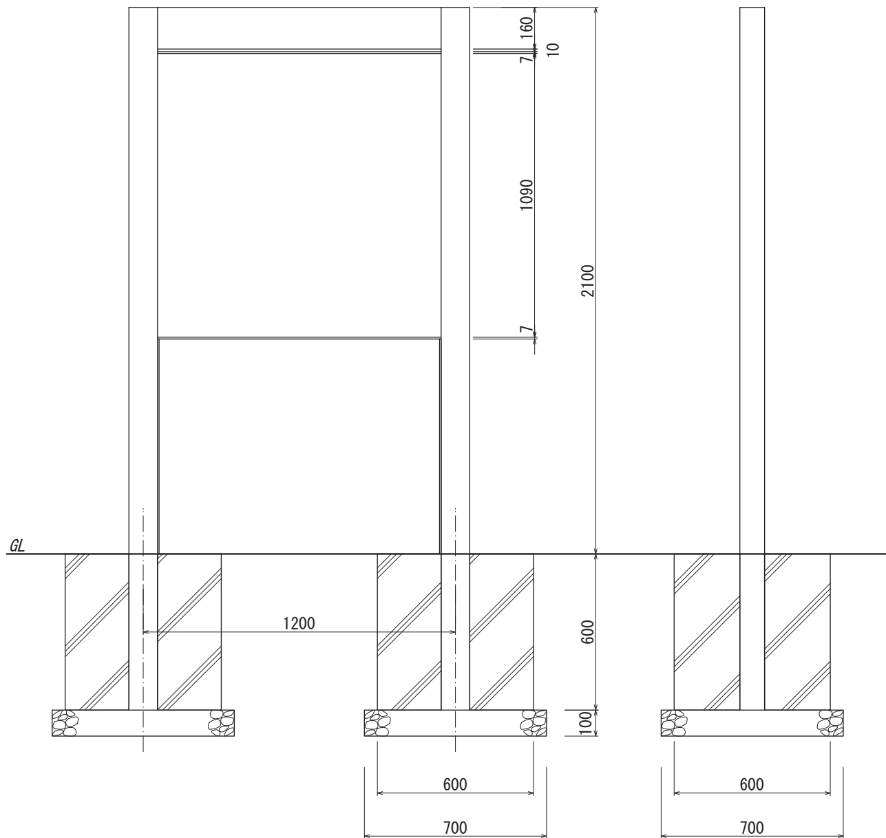
【正面図 S=1:20】
