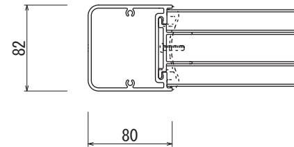
【S支柱】
