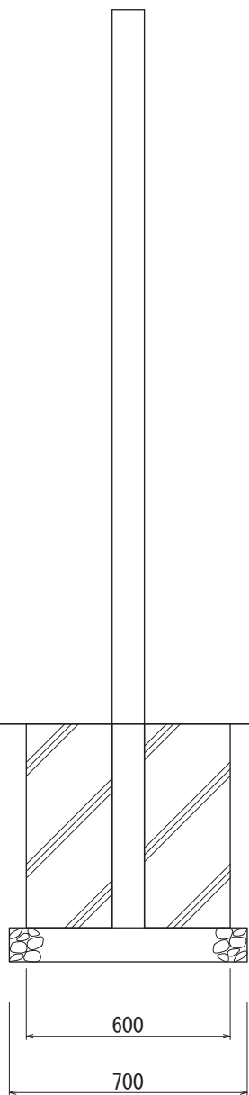
【側面図 S=1:20】
