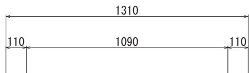
【平面図 S=1:20】
