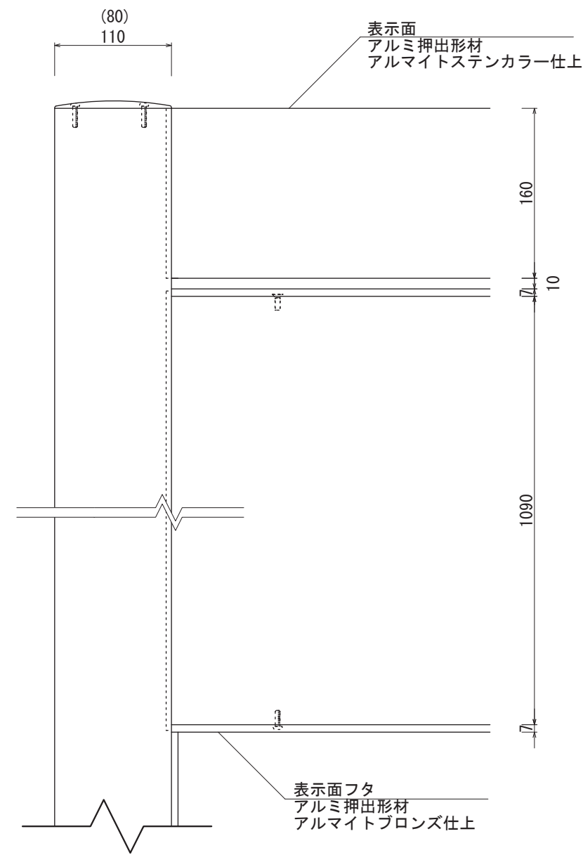
【正面図 S=1:5】
