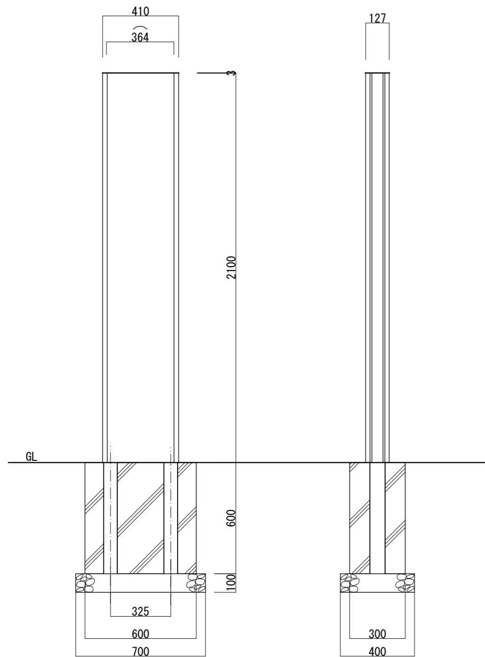
【正面図 S=1:20】
