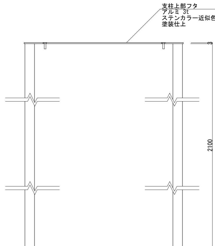
【正面図 S=1:5】
