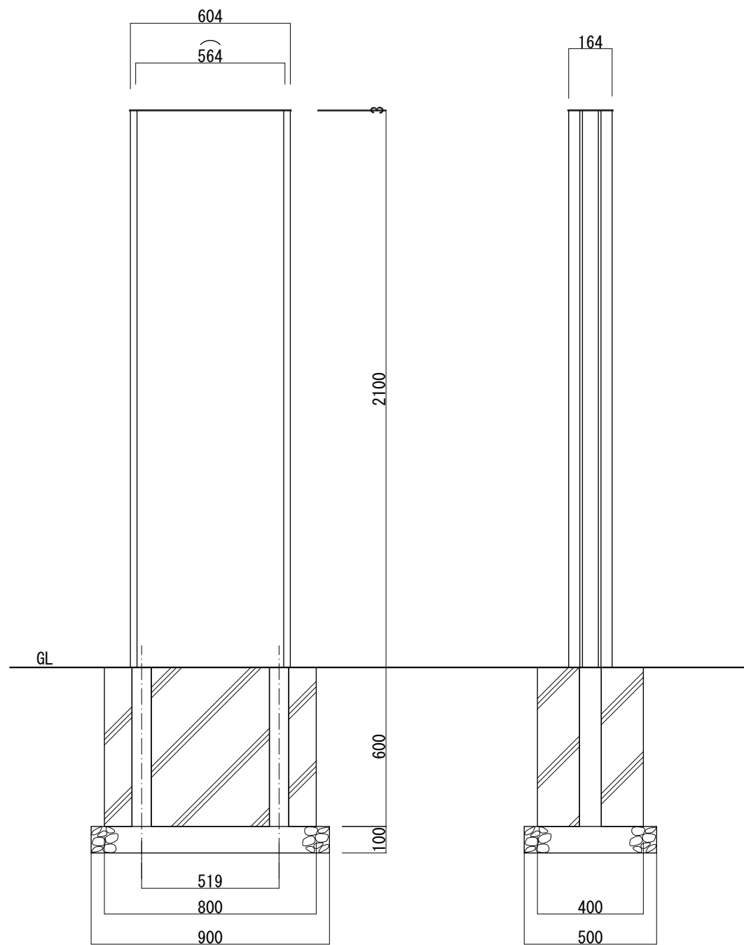
【正面図 S=1:20】
