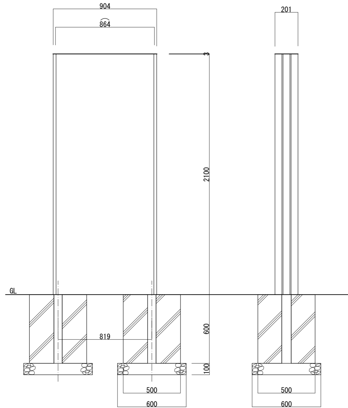
【正面図 S=1:20】
