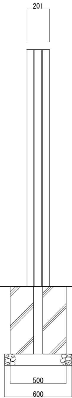
【側面図 S=1:20】
