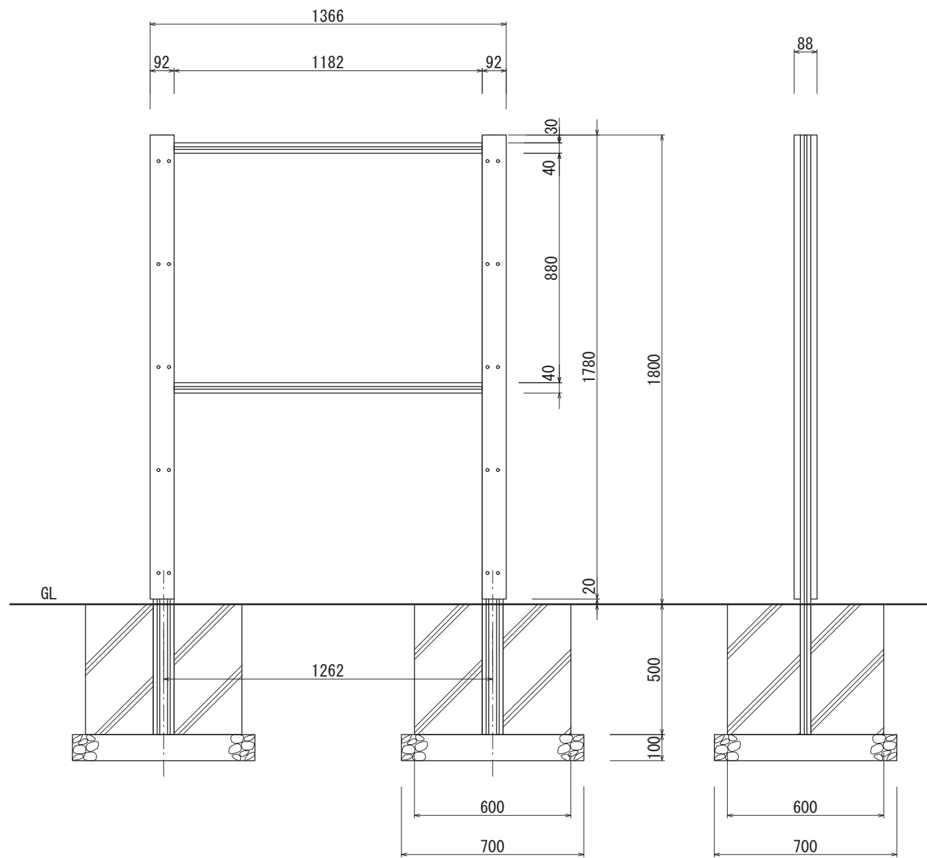
【正面図 S=1:20】
