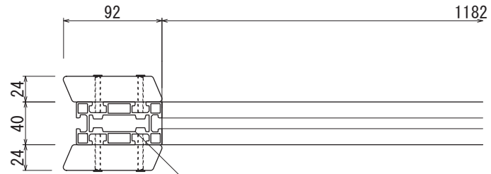
【平面図 S=1:5】
