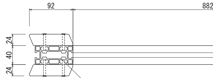
【平面図 S=1:5】
