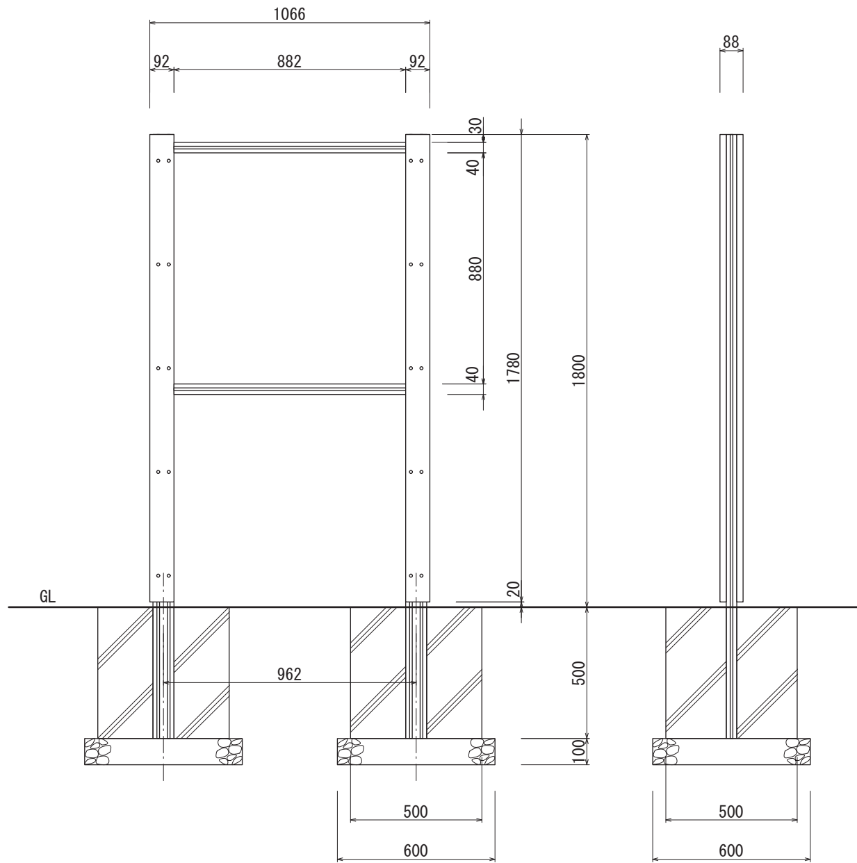
【正面図 S=1:20】
